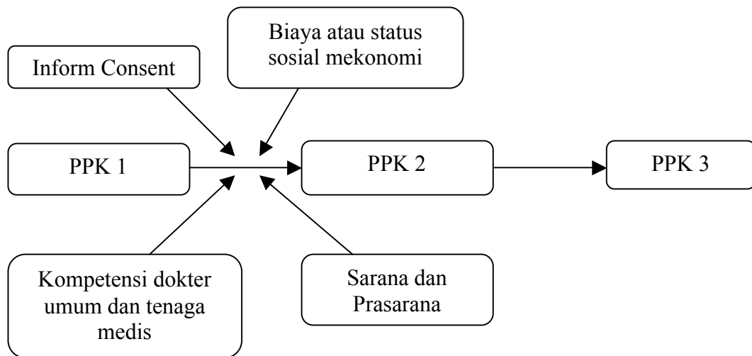
Gambar 2 : Kerangka Teori
