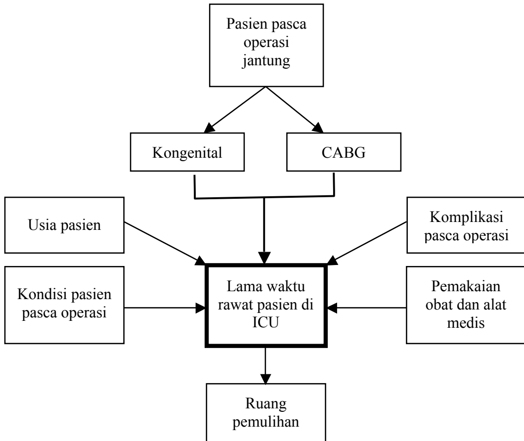
Gambar 10. Kerangka Teori
