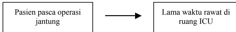
Gambar 11. Kerangka Konsep
