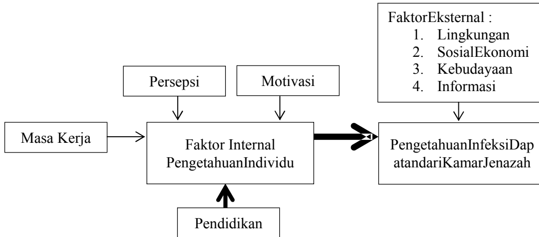
Gambar 2. Kerangka Teori
