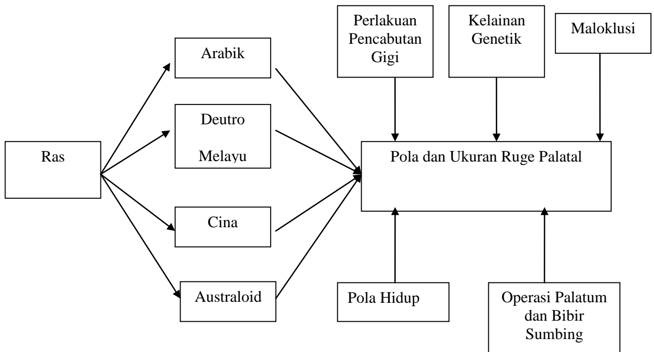
Gambar 5. Kerangka Teori
