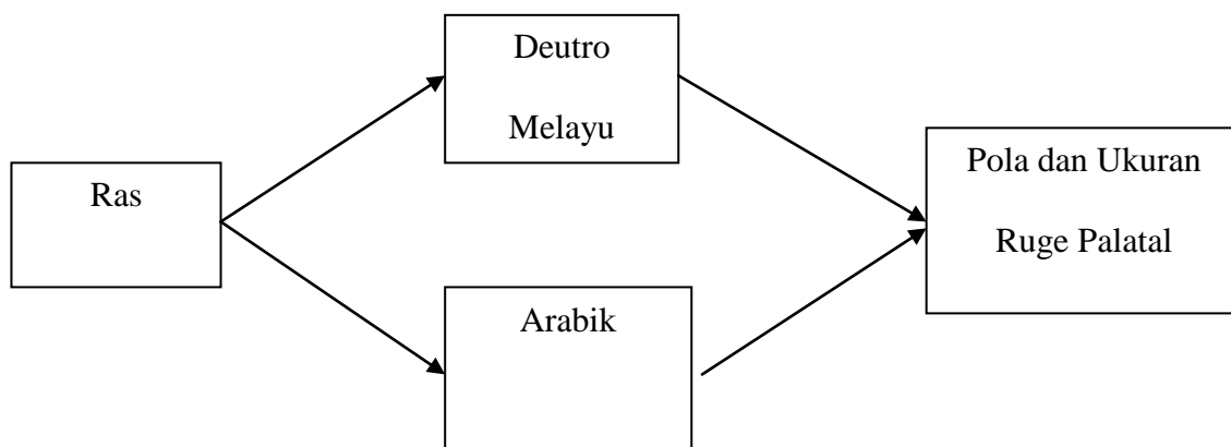
Gambar 6. Kerangka Konsep
