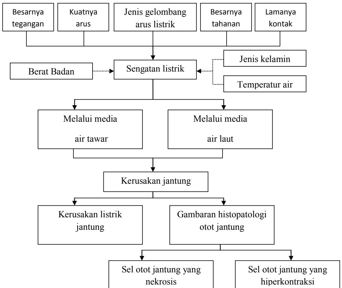
Gambar 3. Kerangka teori
