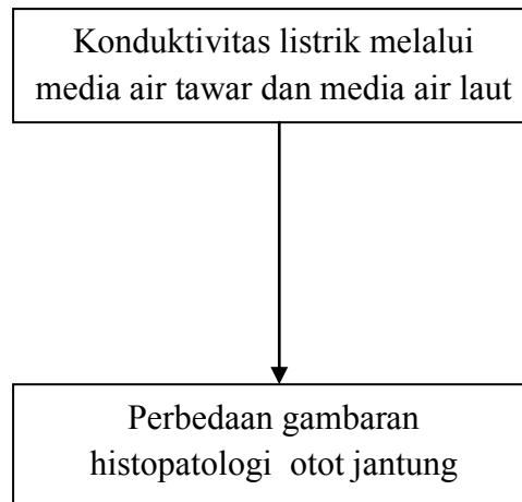
Gambar 4. Kerangka konsep
