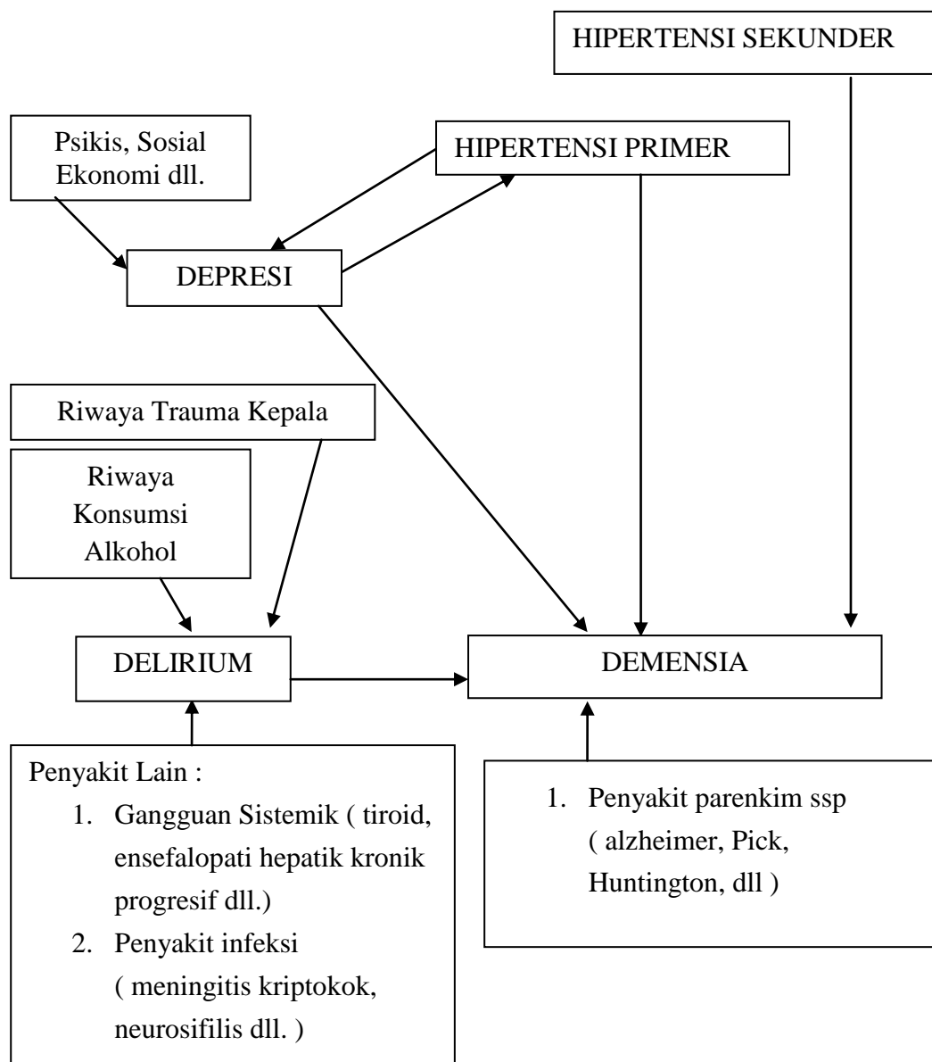
Gambar 1. Kerangka Teori
