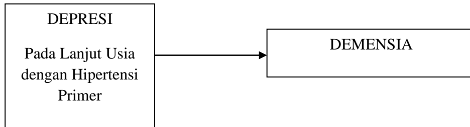
Gambar 2. Kerangka Konsep
