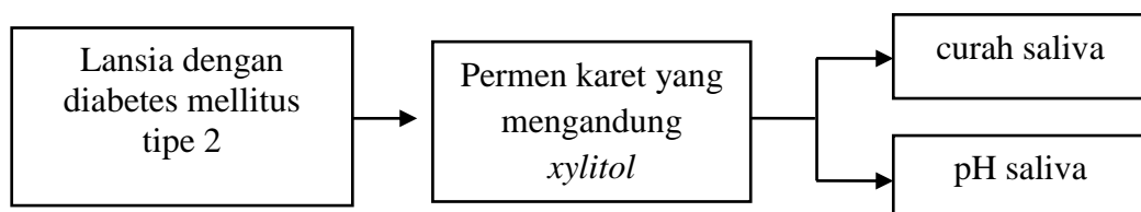
Gambar 5. Kerangka konsep
