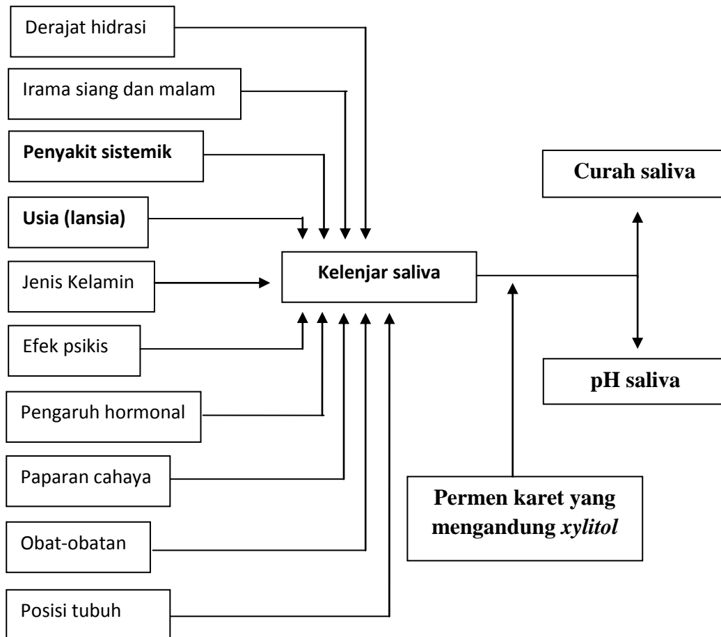
Gambar 4. Kerangka teori
