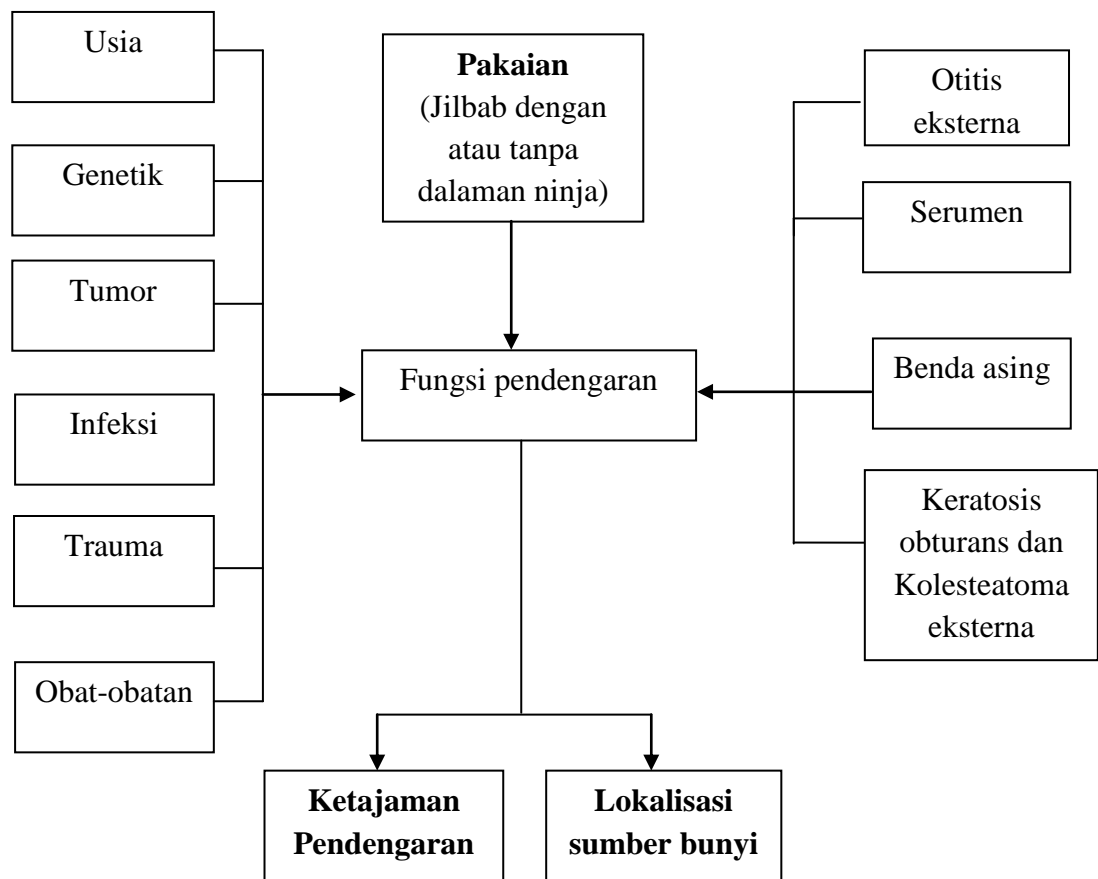
Gambar 13. Kerangka Teori
