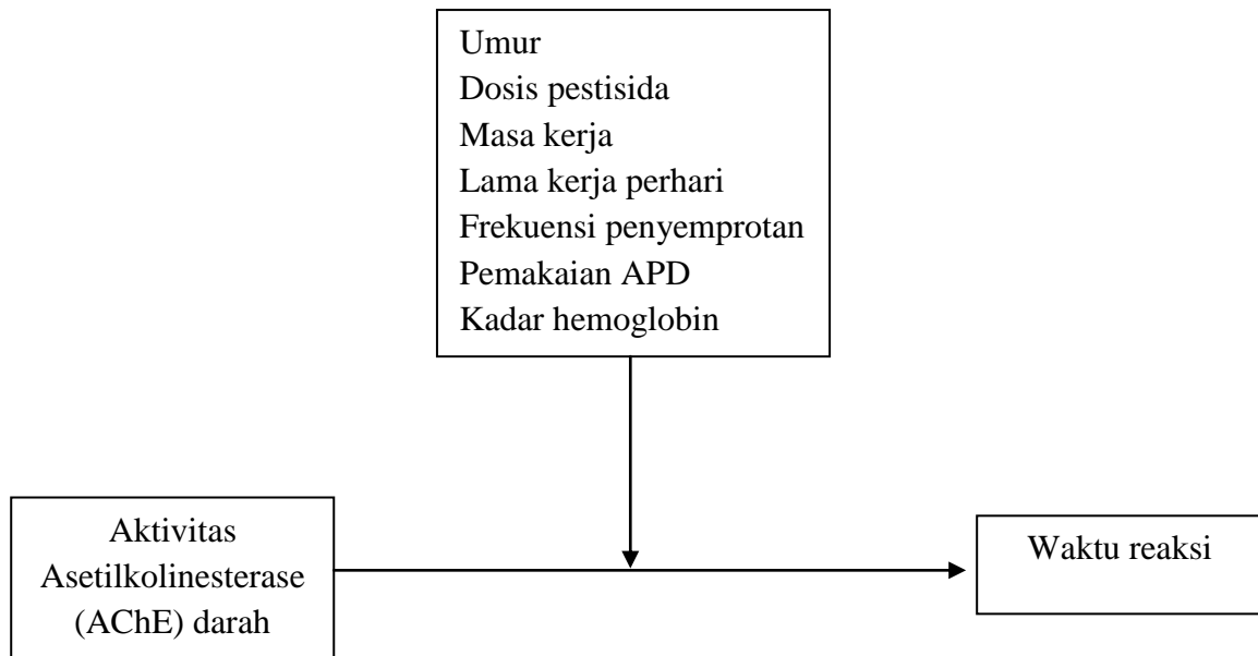
Gambar 4. Kerangka konsep
