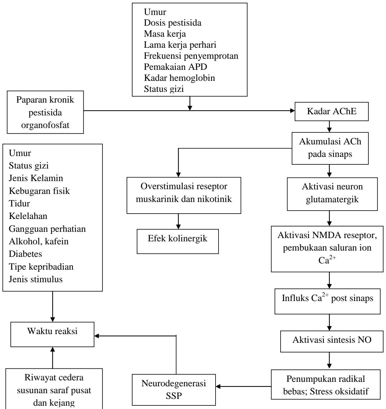
Gambar 3. Kerangka teori
