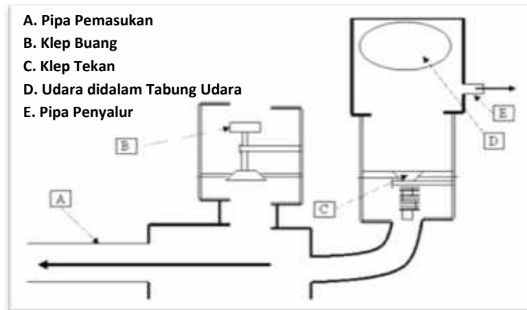
Gambar 2.5 Skema pompa hidram pada tahap pengantar
