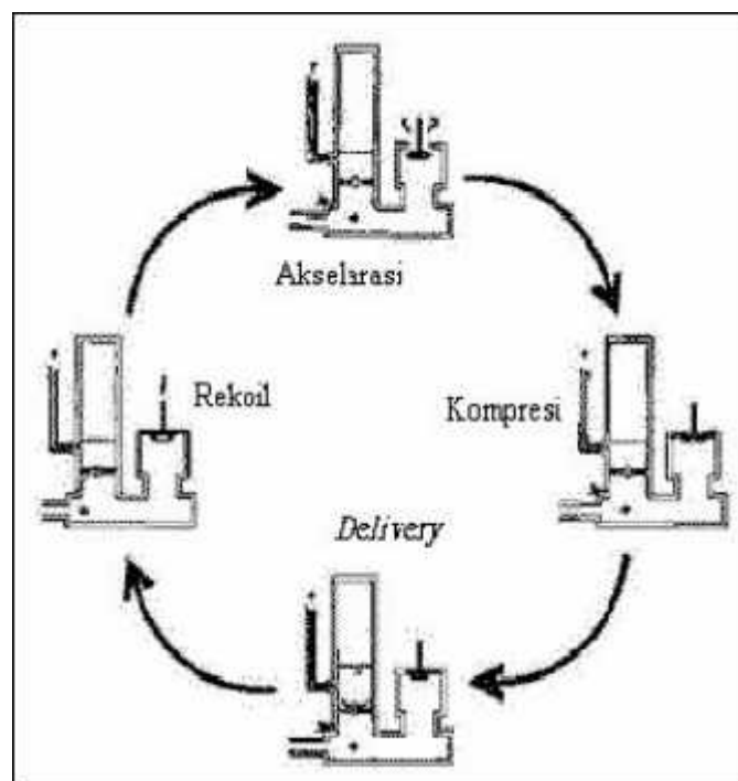
Gambar 2.2 Prinsip kerja pompa hidram
