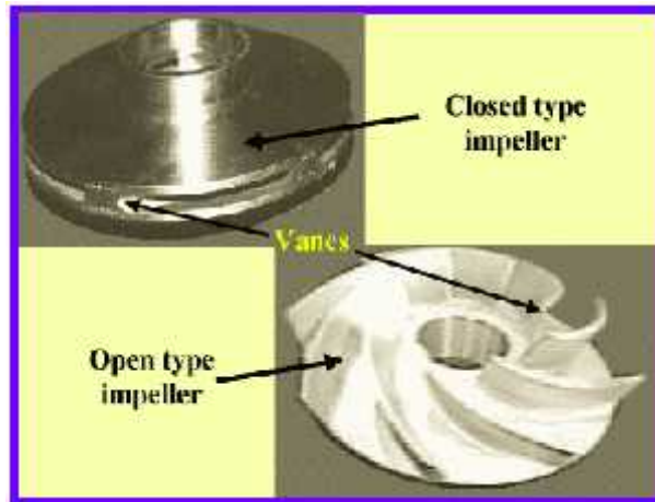
Gambar 2.6 Impeler
