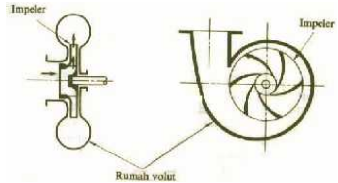
Gambar 2.7 Pompa volut
