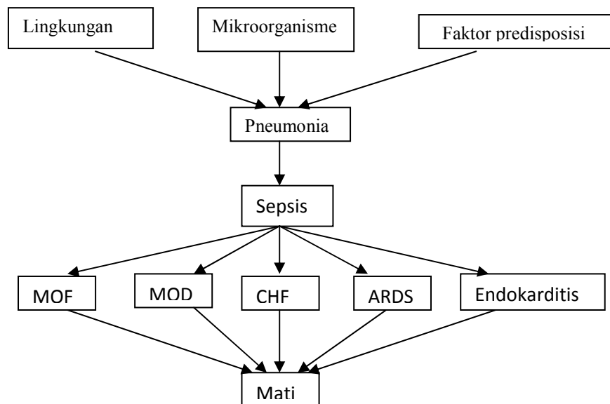
Gambar 2. Kerangka Teori 21
