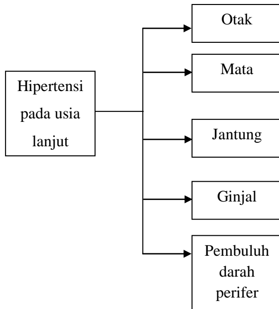
Gambar 6. Kerangka konsep
