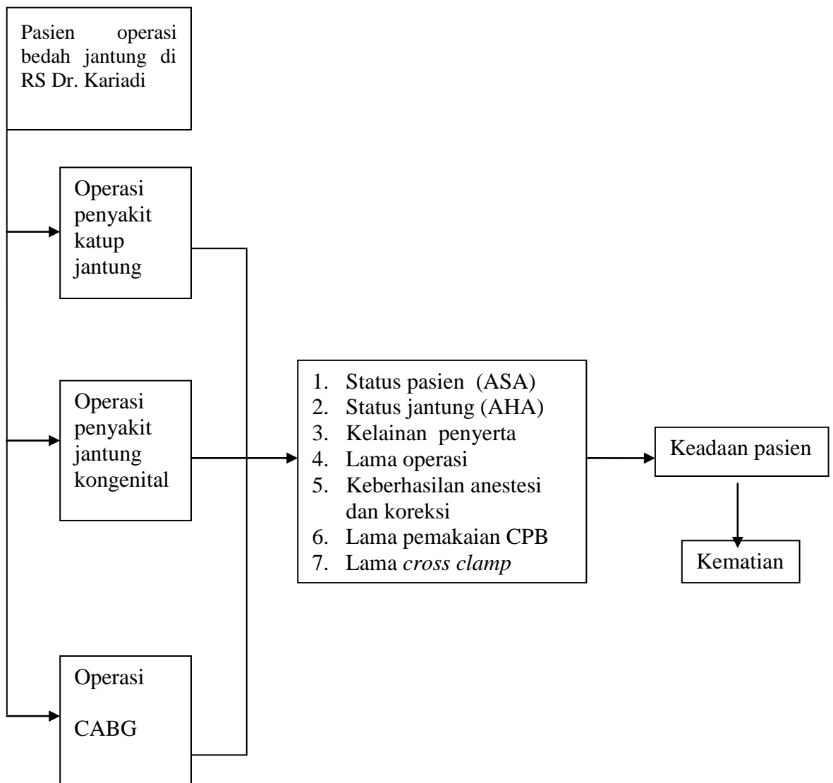
Gambar 5. Kerangka teori
