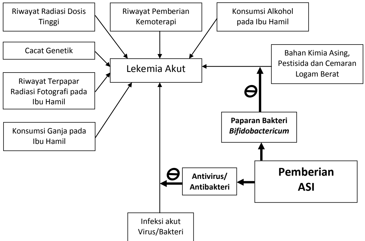
Gambar 1. Kerangka teori
