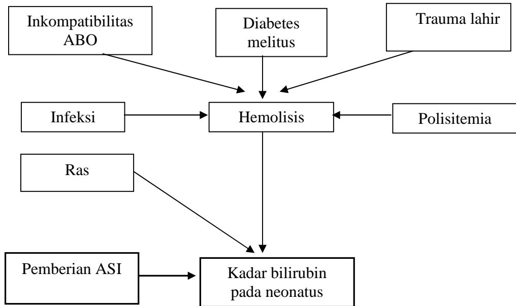
Gambar 1. Kerangka teori
