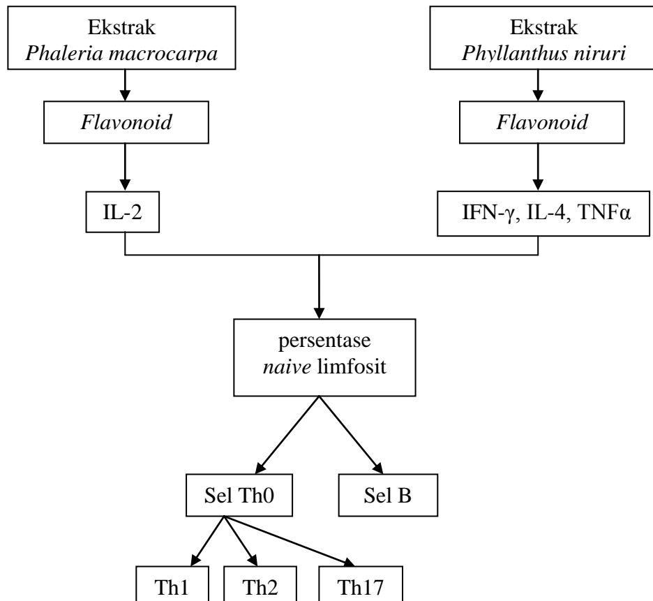
Gambar 5. Kerangka Teori
