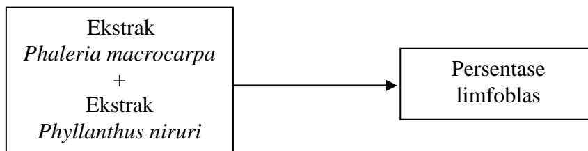
Gambar 6. Kerangka Konsep
