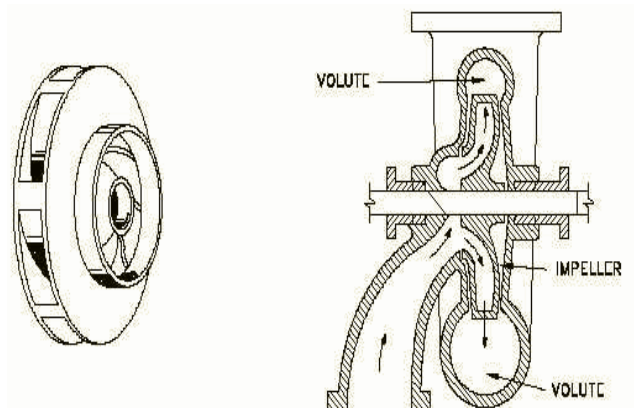
Gambar 2.3 Pompa sentrifugal aliran radial
