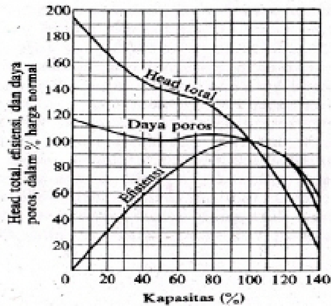
Gambar 2.15 Kurva karakteristik pompa aliran campuran
