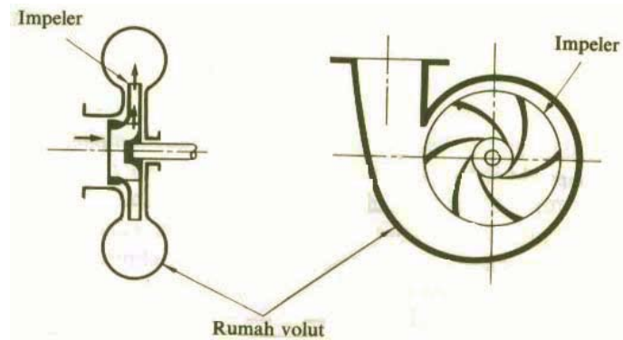
Gambar 2.7 Pompa volut
