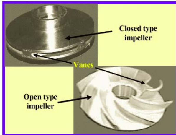
Gambar 2.6 Impeler
