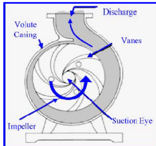
Gambar 2.1 Lintasan Aliran Cairan Pompa Sentrifugal.
