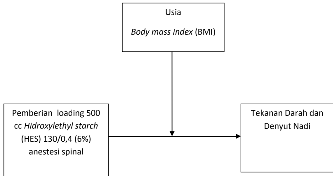
Gambar 3.2 kerangka konsep
