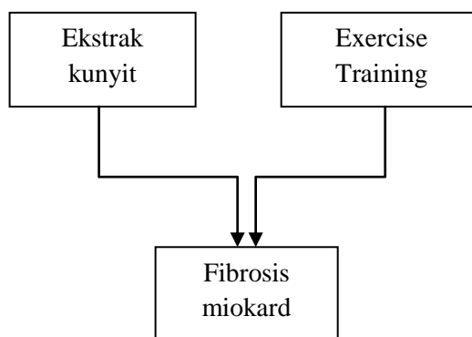
Gambar 2. Kerangka Konsep
