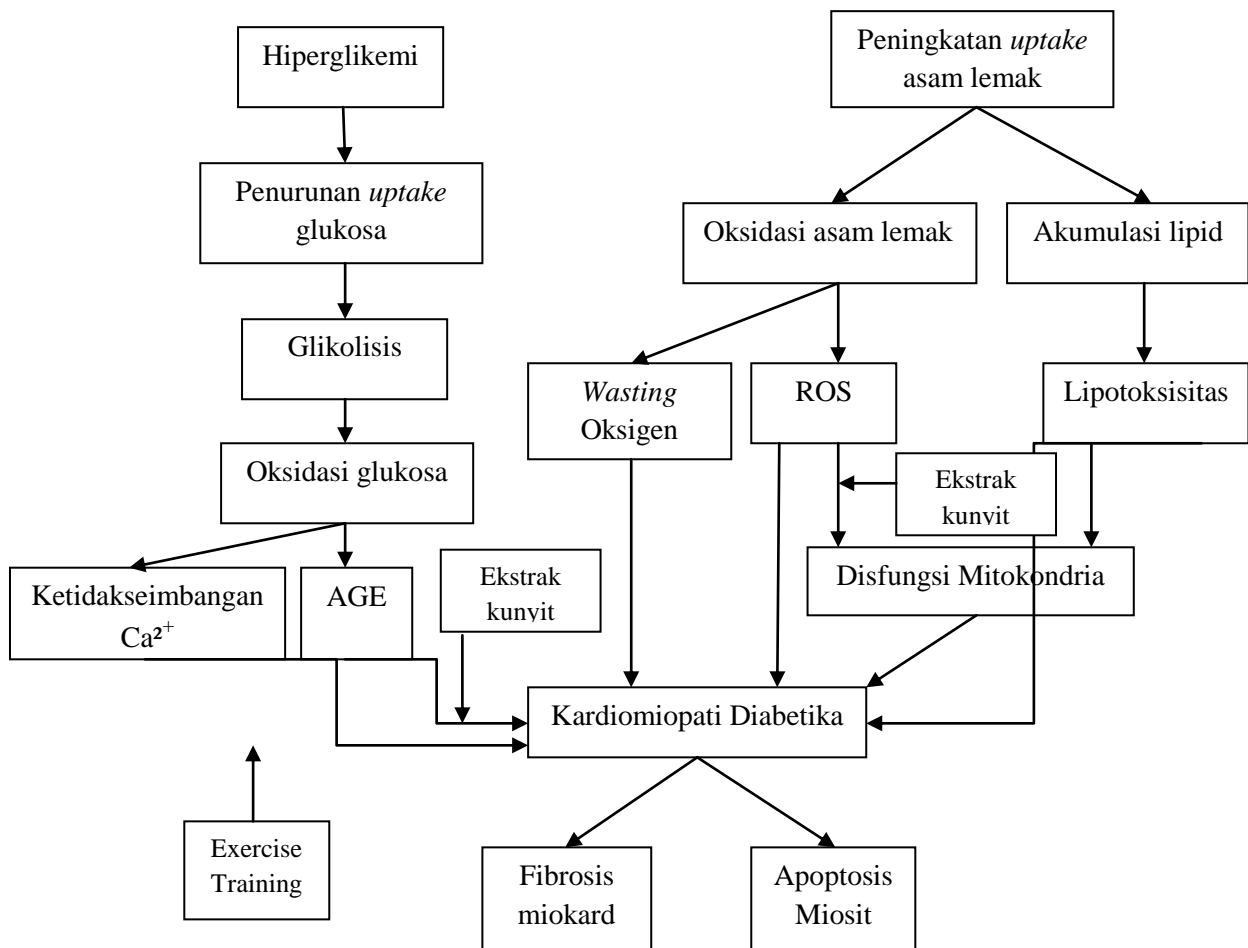
Gambar 1. Kerangka Teori
