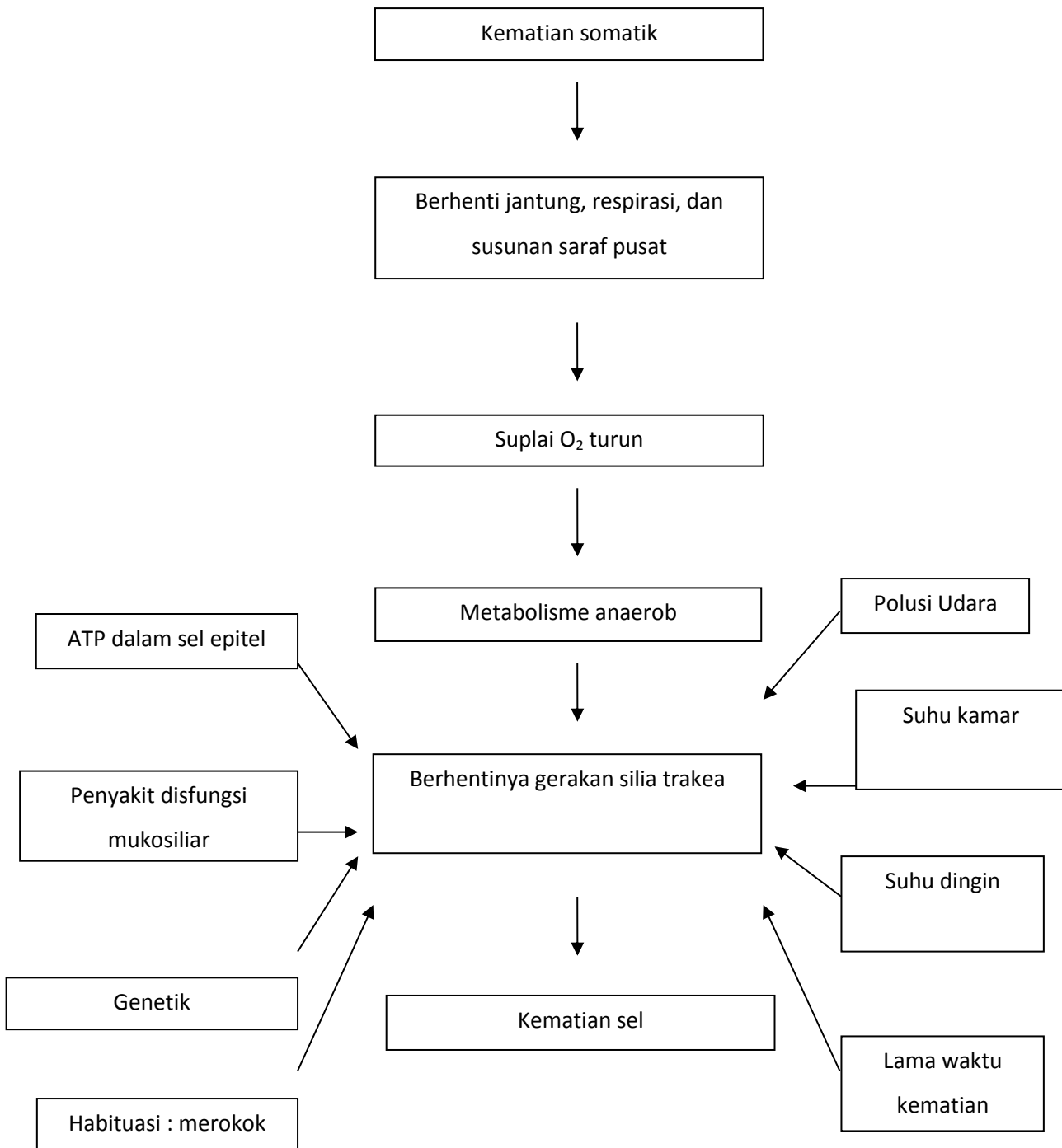
Gambar 4. Kerangka Teori
