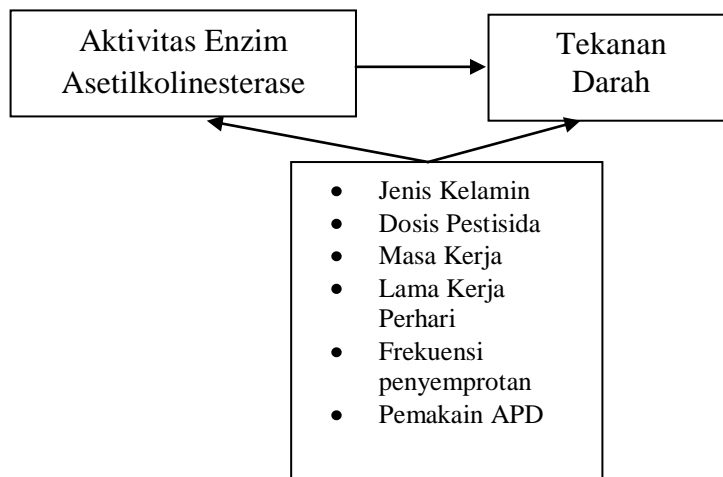
Gambar 5. Kerangka Konsep
