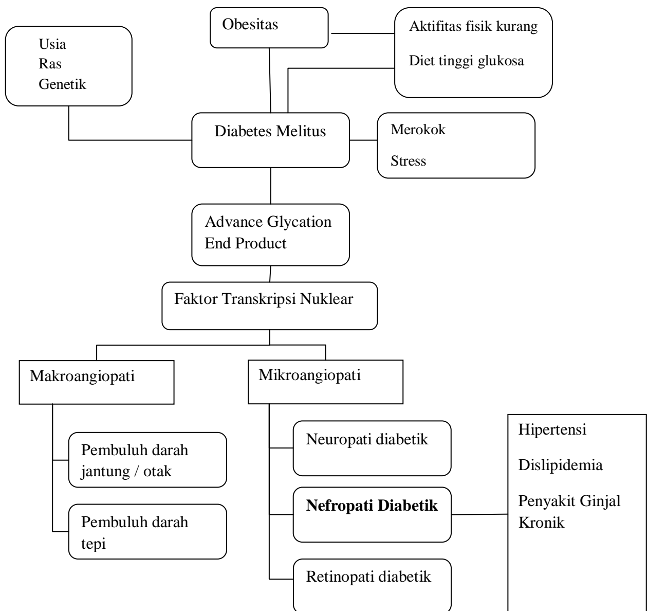
Gambar 8 : Kerangka Teori
