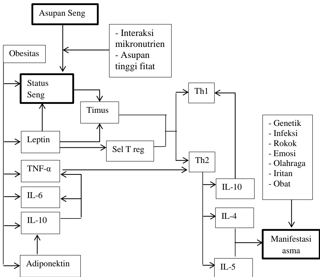
Gambar 3. Kerangka Teori
