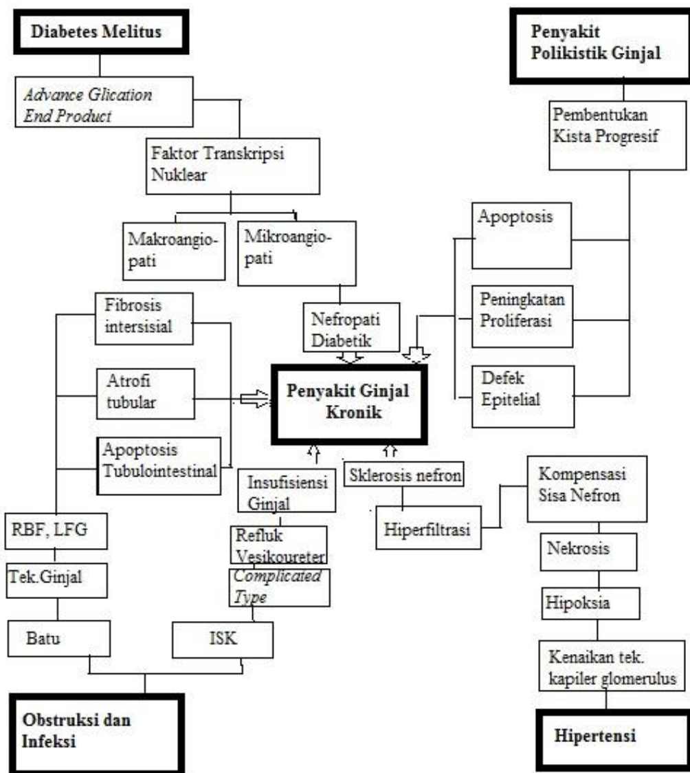
Gambar 1 : Kerangka Teori
