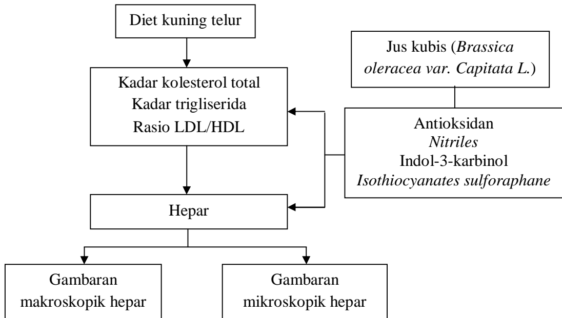
Gambar 1. Kerangka teori
