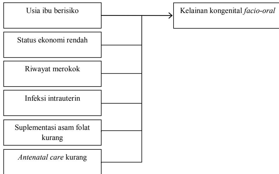
Gambar 15. Kerangka Konsep
