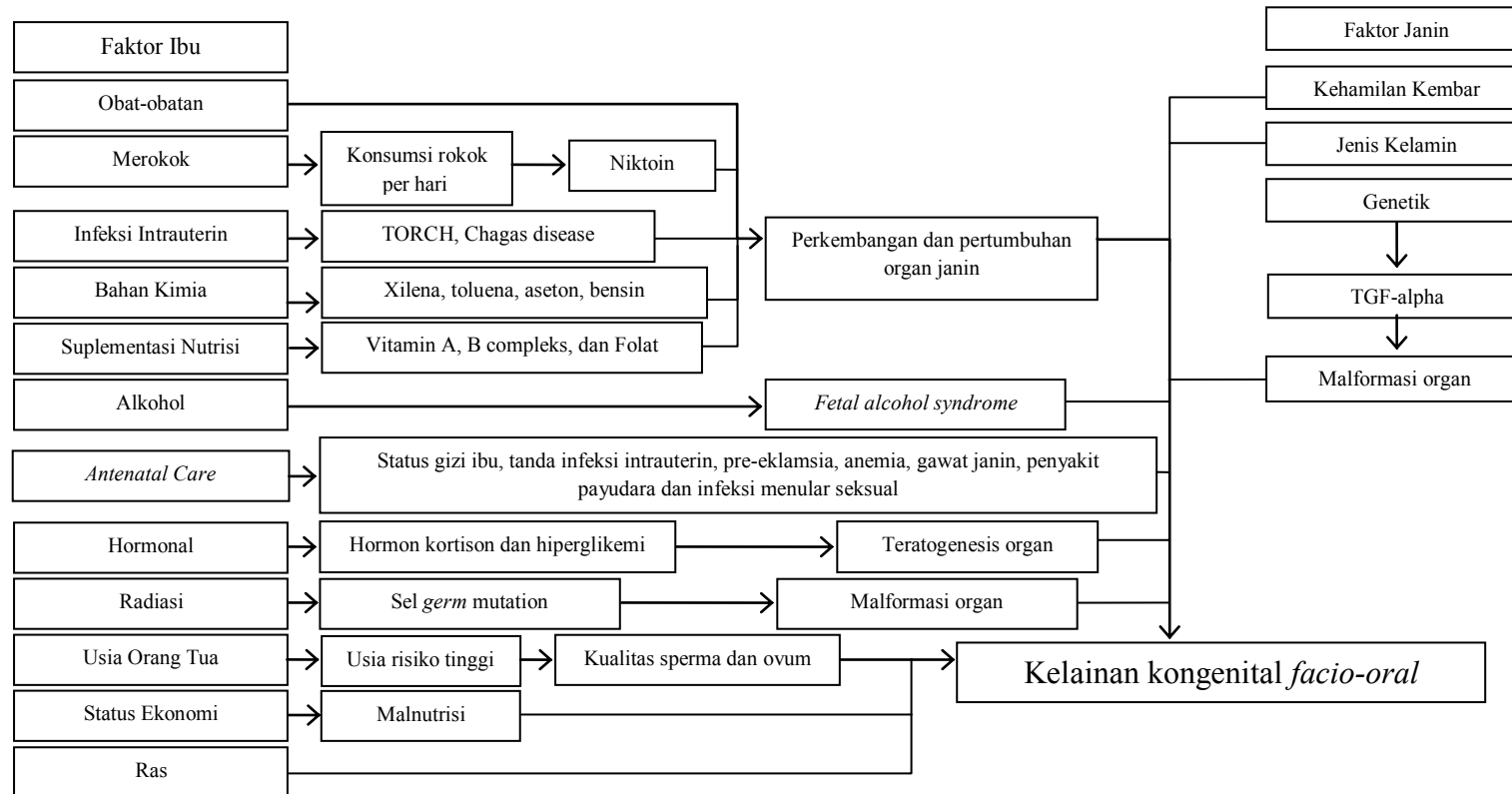
Gambar 14. Kerangka Teori
