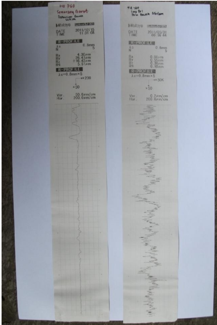
Lampiran 5: Grafik kekasaran permukaan bawah HQ 760 A
