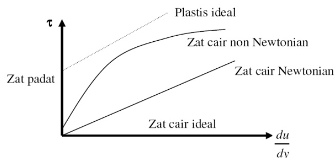
Grafik 2.2. Hubungan Tegangan Geser dan Gradien Kecepatan (Darmadi, 2011)
