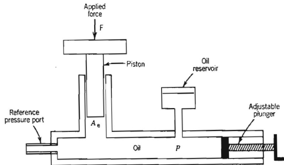
Gambar 2.3. Design Alat Pengukur Tekanan Secara Teori
