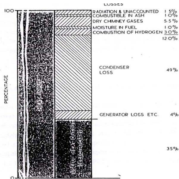
Gambar 2.6 Korelasi Input, Output dan Losses terhadap efisiensi
