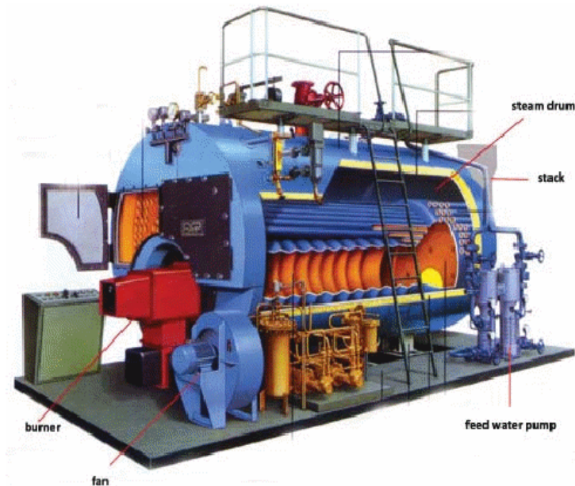
Gambar 2.1 Ketel Pipa Api (Omnicol)
