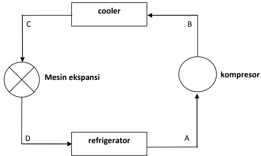
Gambar 2.8. Sistem refrigerasi udara (Sunyoto,2010)
