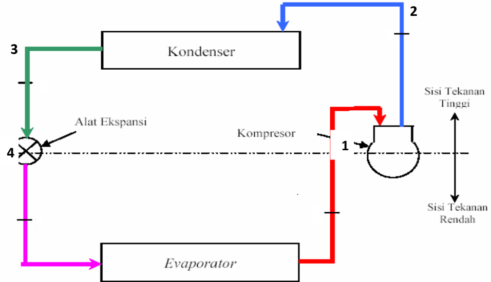
Gambar 2.6. Sistem refrigerasi kompresi uap(Sunyoto,2010)
