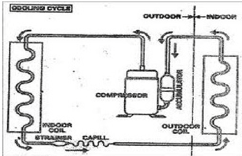
Gambar 2.1. Prinsip Kerja Mesin Pendingin Ruangan
