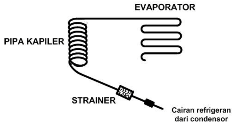
Gambar 2.2. Pipa Kapiler(Sunyoto,2010)
