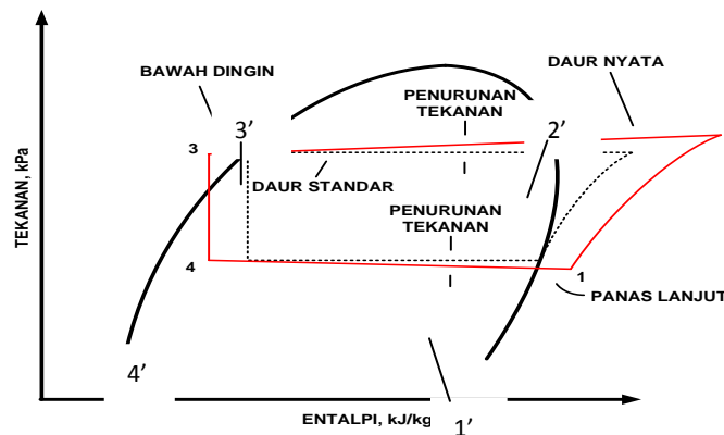
Gambar 2.5. Perbandingan siklus aktual dan siklus standar (Sunyoto, 2010)
