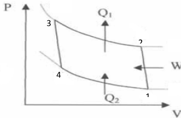
Gambar 2.3. Daur refrigerasi carnot(Sunyoto,2010)
