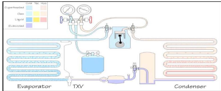
Gambar 2.9. Pemasangan Manifold untuk pengisian
