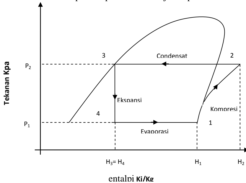
Gambar 2.4. Diagram tekanan entalpi siklus kompresi uap standar (Sunyoto,2010)
