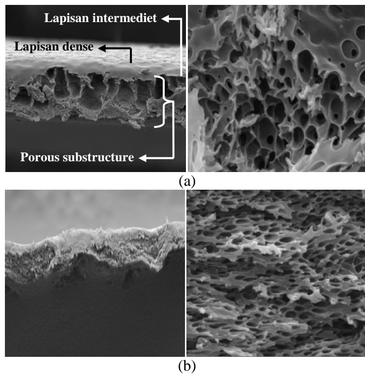
Gambar 9 : Penampang melintang membran pada suhu pemanasan : (a) 60 °C dan (b) 70 °C
