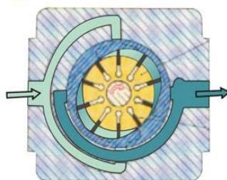
Gambar 2.6 Pompa Sirip Burung
