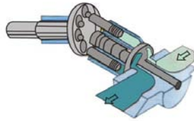
Gambar 2.7 Pompa Torak Aksial
