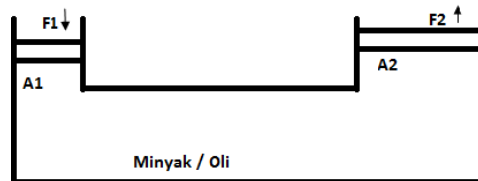
Gambar 2.1 Minyak Dalam Pipa Menurut Hukum Pascal
