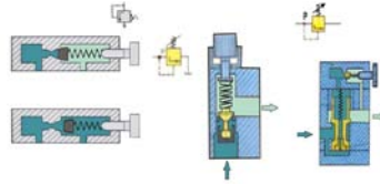
Gambar 2.10 Macam-macam Katup Pengatur Tekanan
