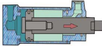
Gambar 2.13 Kontruksi Silinder Kerja Penggerak Ganda
