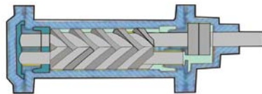
Gambar 2.9 Pompa Sekrup
