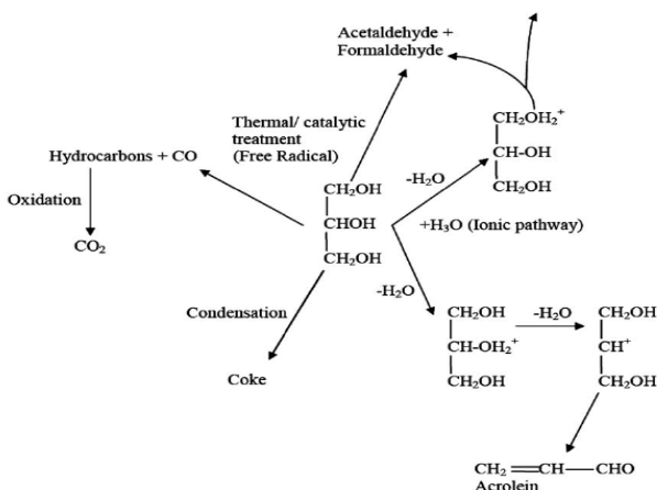
Gambar 5. Kemungkinan-Kemungkinan Terbentuknya Produk (Pathak, dkk., 2009)
