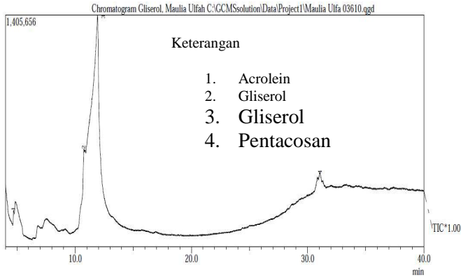
Gambar 4. Hasil Analisa GC-MS
