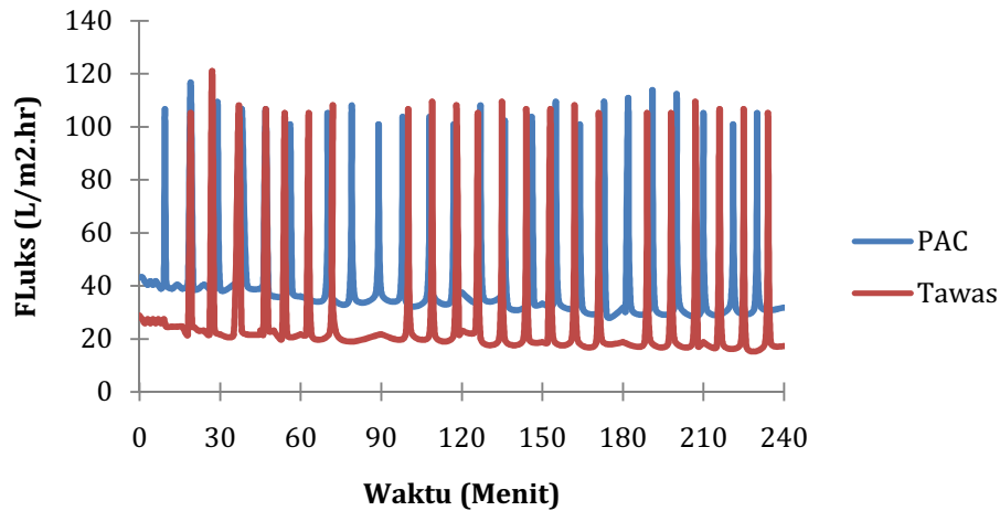
Gambar 4.3 Karakteristik Penurunan Fluks pada Membran Ultrafiltrasi dengan Menggunakan Umpan Hasil Proses Dissolved Air Flotation
