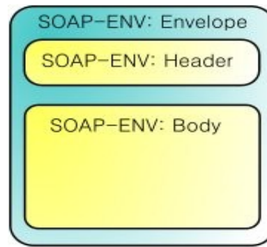
Gambar 1 Struktur SOAP[13]
