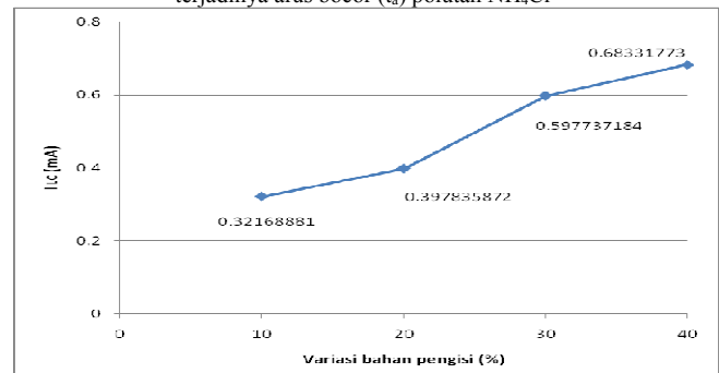
Gambar 4.6 Grafik hubungan komposisi pengisi (%) dengan arus bocor rata-rata ( I_{rc} ) polutan \text{NH}_4\text{Cl}
