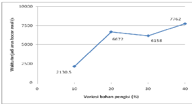
Gambar 4.7 Grafik hubungan komposisi pengisi (%) dengan waktu terjadinya arus bocor ( t_0 ) polutan pantai
