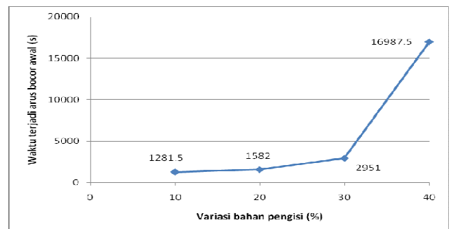
Gambar 4.5 Grafik hubungan komposisi pengisi (%) dengan waktu terjadinya arus bocor ( t_b ) polutan \text{NH}_4\text{Cl}
