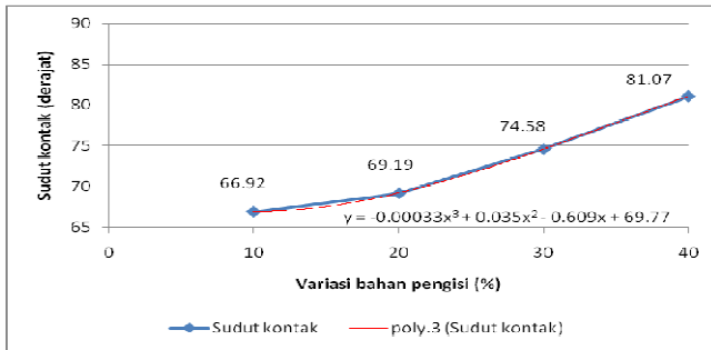
Gambar 4.3 Grafik hubungan sudut kontak dengan variasi bahan pengisi polutan Pantai
