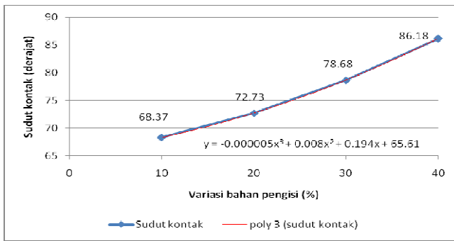
Gambar 4.2 Grafik hubungan sudut kontak dengan variasi bahan pengisi polutan \text{NH}_4\text{Cl}
