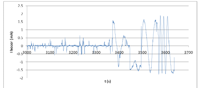
(c) Gelombang arus bocor saat kegagalan isolasi pada t_b = 3372 s
