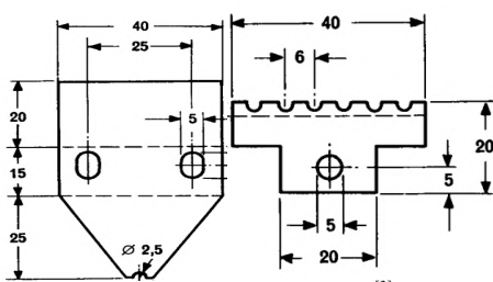
Gambar 3.2 Bentuk elektroda [3]
