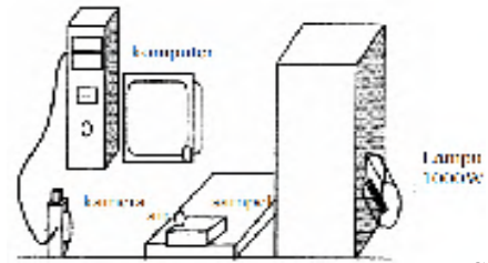
Gambar 3.4 Rangkaian pengukuran sudut kontak [11,19]
