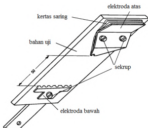
Gambar 3.3 Pemasangan elektroda [3]
