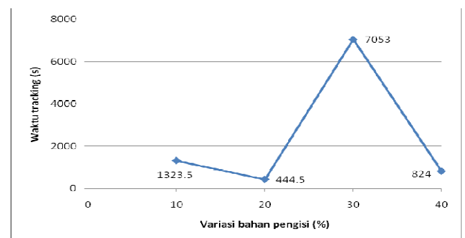
Gambar 4.9 Hubungan komposisi bahan (%) terhadap waktu tracking ( t_{tracking} ) polutan NH_4Cl
