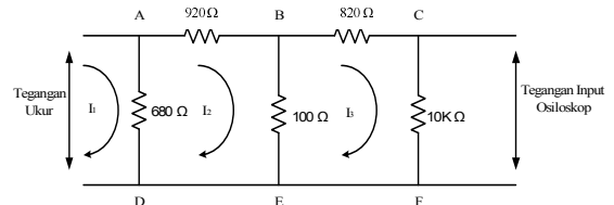
Gambar 3.6 Rangkaian pembagi tegangan
