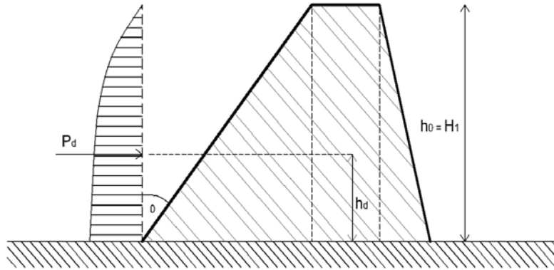
Gambar 2.16 Gaya Tekan Air Dinamik
