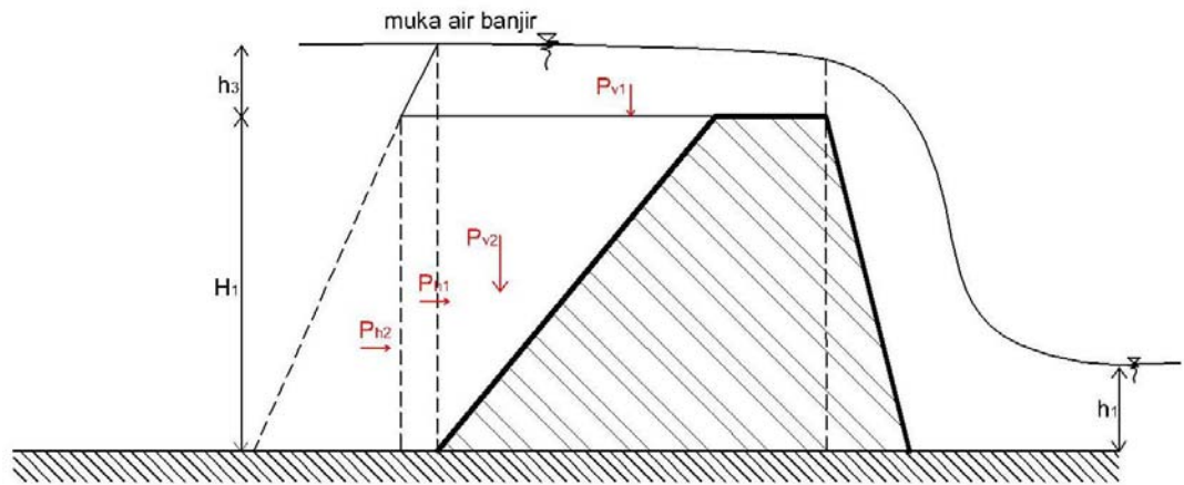
Gambar 2.12 Gaya Tekan Air Statik
