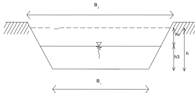
b. Potongan Melintang Pelimpah
