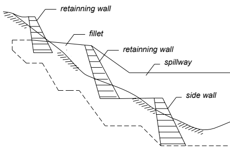
Gambar 2.22 Penetrasi Sayap
