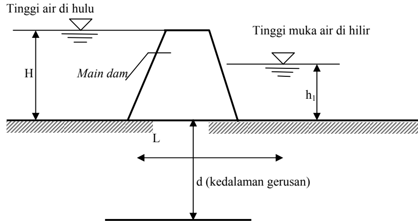
Gambar 2.19 Pemeriksaan Bahaya Piping
