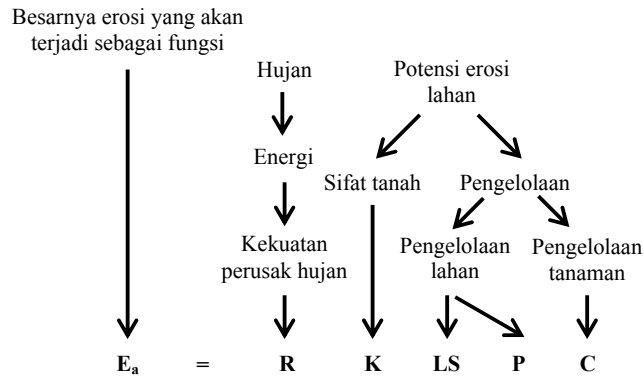
Gambar 2.2 Skema Persamaan USLE (Suripin 2004)
