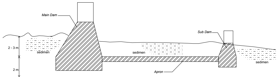
Gambar 2.18 Penetrasi Pondasi pada Main Dam
