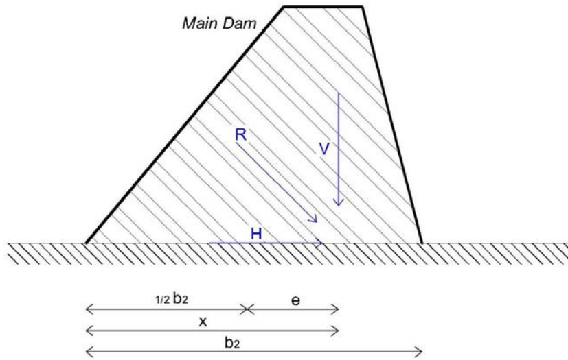
Gambar 2.17 Resultan Gaya pada Main Dam
