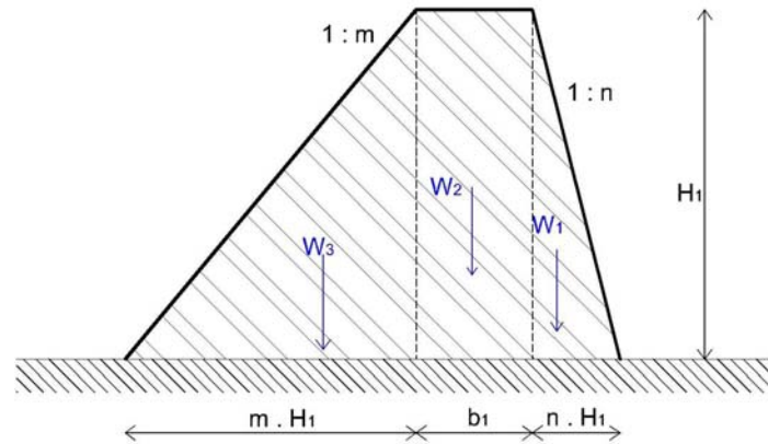
Gambar 2.11 Gaya Berat Sendiri Main Dam
