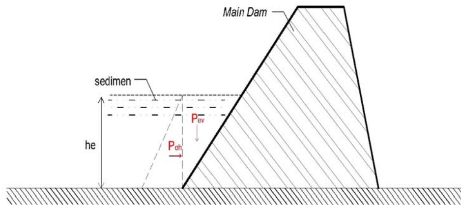
Gambar 2.13 Gaya Tekan Akibat Sedimen
