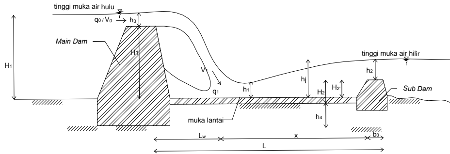
Gambar 2.23 Letak Sub Dam
