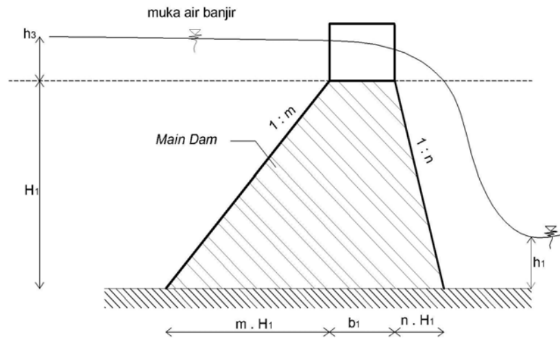
Gambar 2.10 Perencanaan Main Dam
