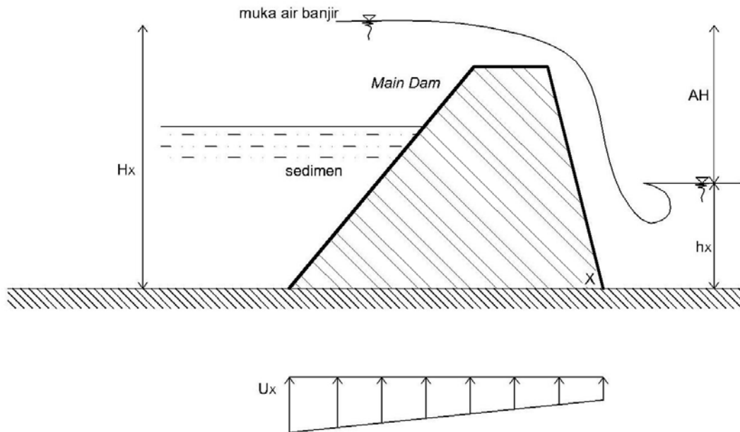
Gambar 2.14 Gaya Angkat pada Main Dam
