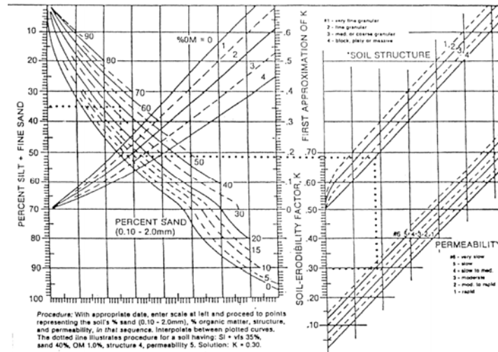
Gambar 2.3 Nomograf K yang Dikembangkan Wischmeier (Asdak 1995)
