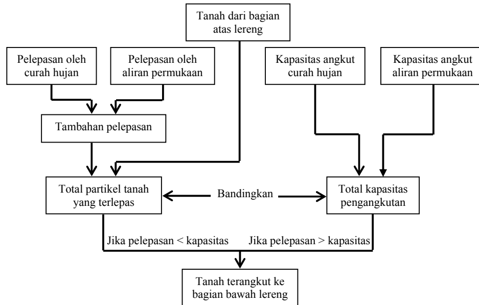
Gambar 2.1 Bagan Alir Model Proses Erosi Lahan oleh Air (Suripin 2004)
