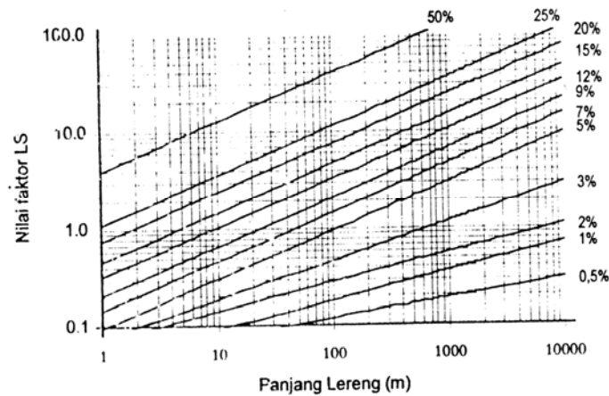
Gambar 2.4 Nomograf untuk Menghitung Faktor LS (Suripin 2004)
