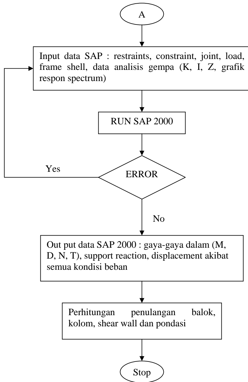
Gambar 3.2 Bagan alir perhitungan mekanika portal 3D
