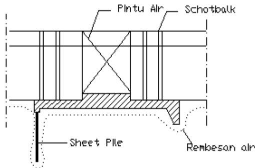
Gambar 2.21 Rembesan Air pada Pintu Air
