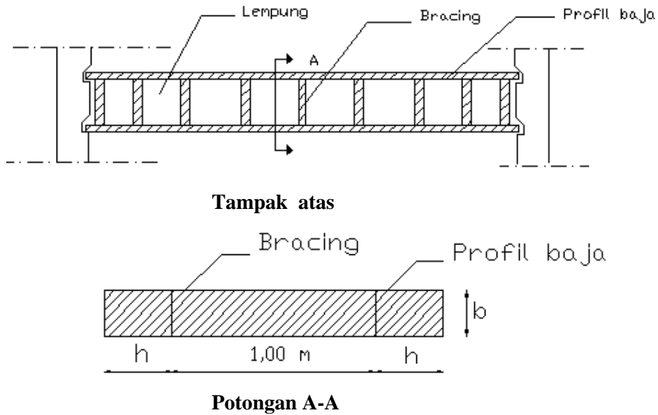
Gambar 2.8. Balok Bracing pada Schotbalk
