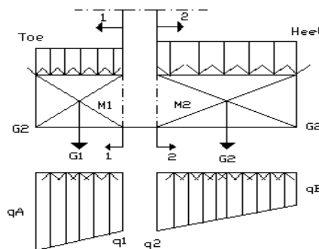
Gambar 2.20 Gaya yang Bekerja pada Bagian Tapak
