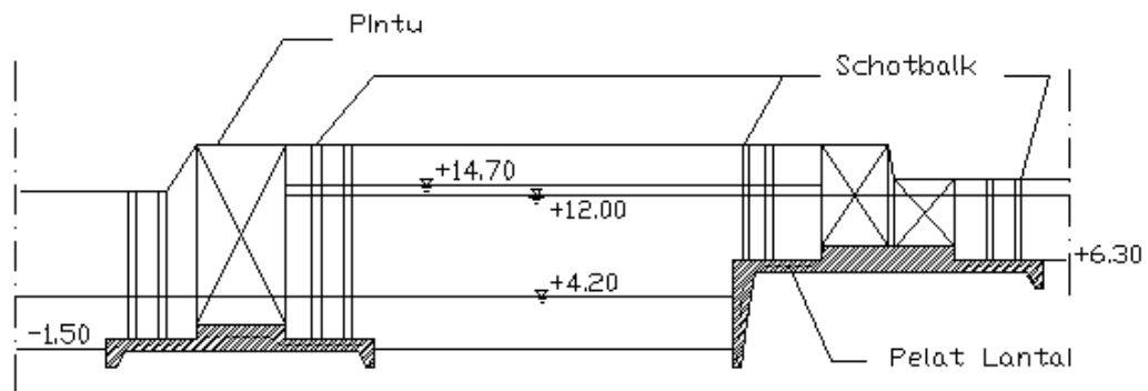
Potongan I-I
