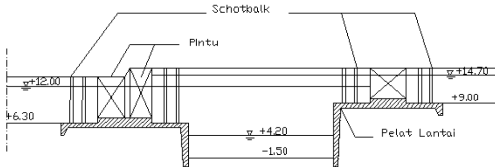
Potongan II-II
