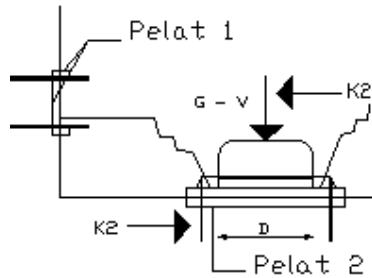
Gambar 2.17 Engsel Bawah
