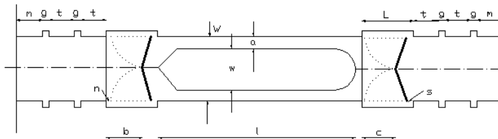
Gambar 2.3 Kelonggaran Memanjang Kapal
