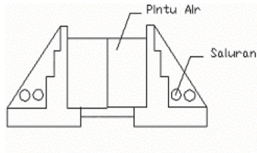
Gambar 2.24 Saluran Pengisian/ Pengosongan pada Dinding
