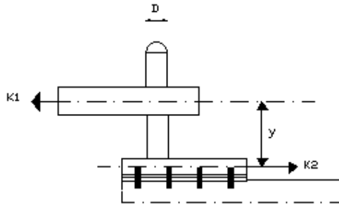
Gambar 2.14 Engsel Atas
