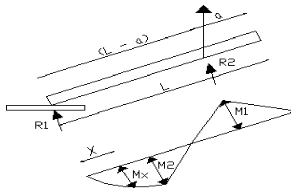
Gambar 2.22 Kondisi Saat Pemancangan Tiang pancang
