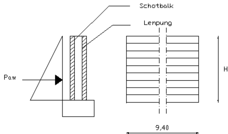
Gambar 2.6. Tekanan Hidrostatis pada Schotbalk
