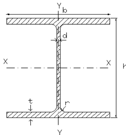
Gambar 2.7. Penampang Profil Baja
