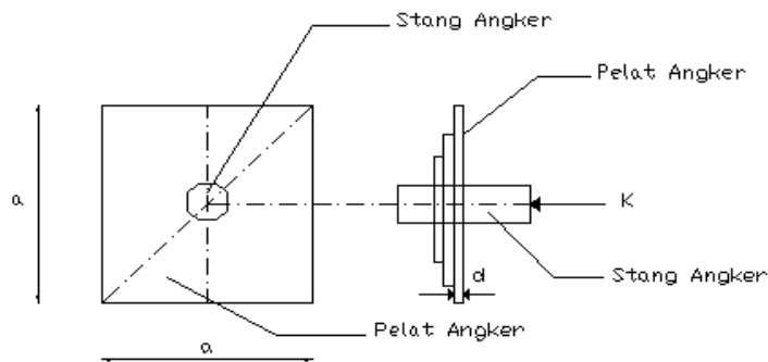
Gambar 2.16 Pelat Angker
