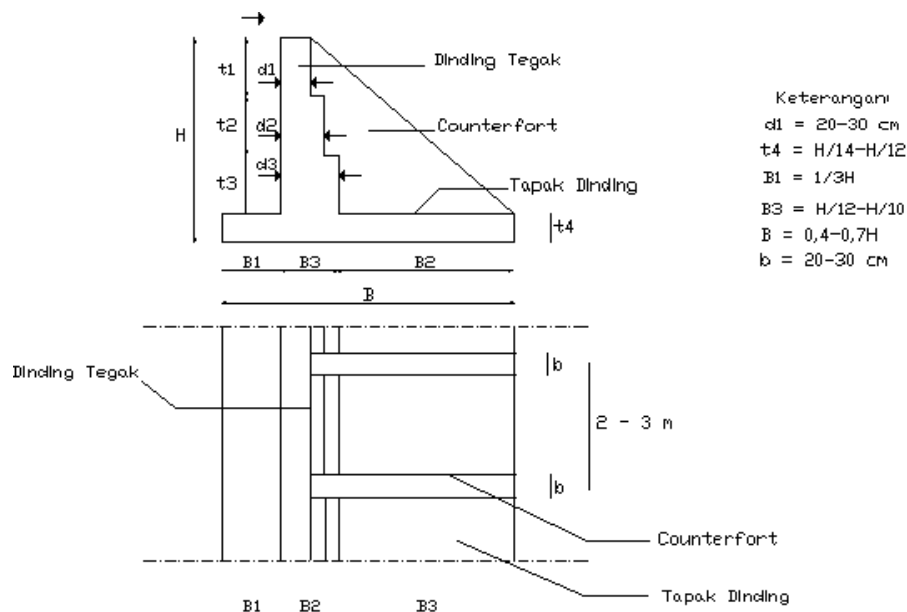
Gambar 2.19 Bentuk Rencana Dinding Kolom
