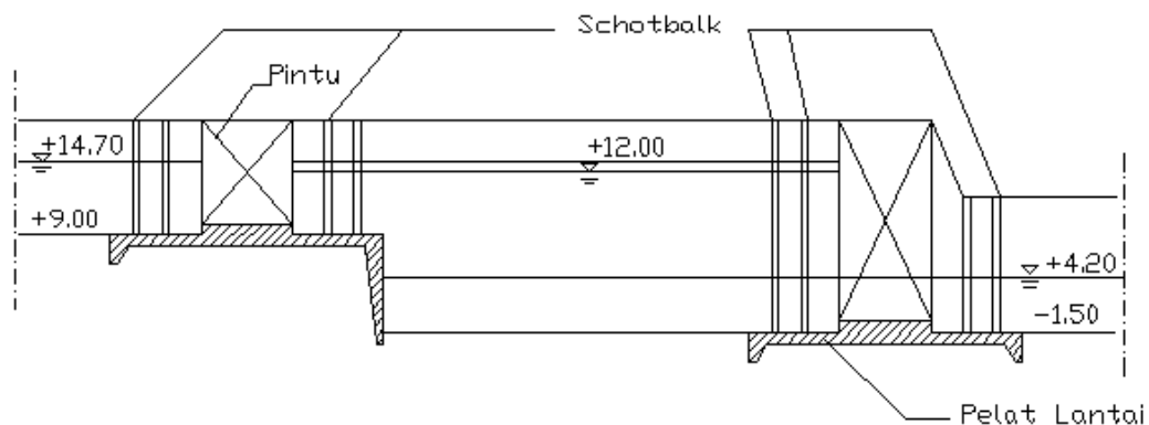
Potongan III-III
