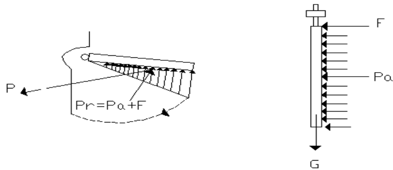
Gambar 2.23 Pengoperasian Pintu Gerbang
