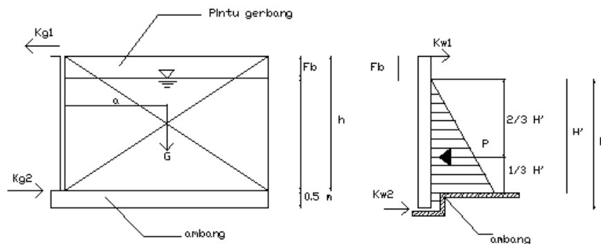
Gambar 2.13. Pembebanan pada Engsel Pintu Gerbang
