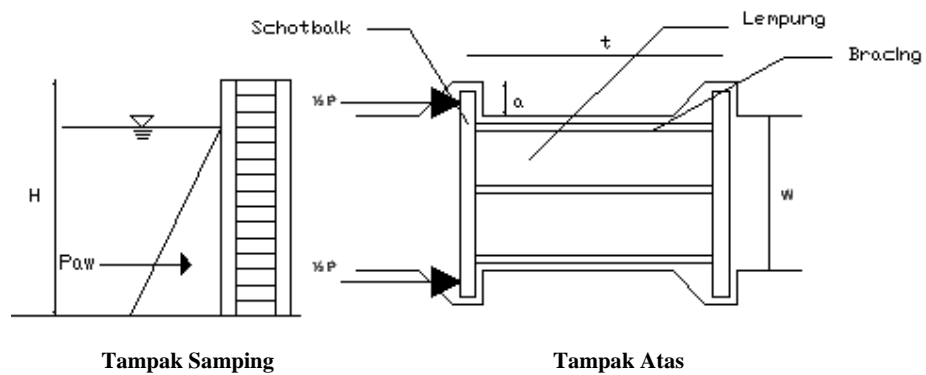
Gambar 2.10. Bidang Geser Dinding Penahan Schotbalk
