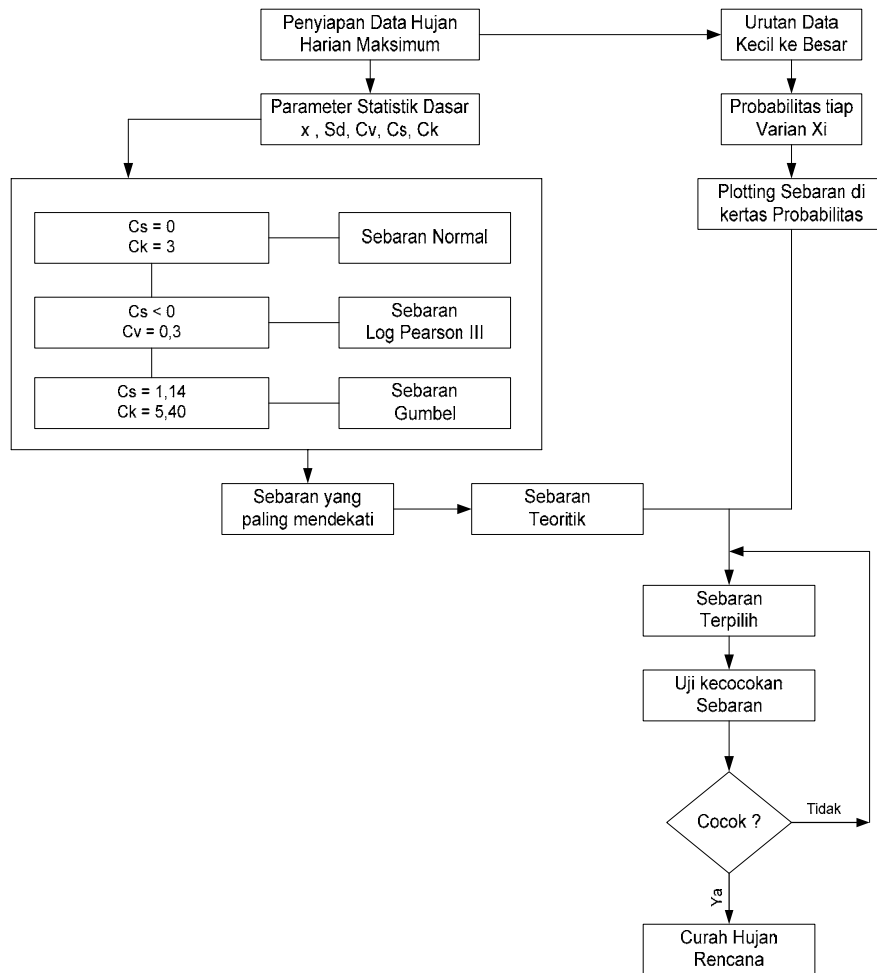
Gambar 2.12 Skema Analisis Frekuensi Hujan Rencana
