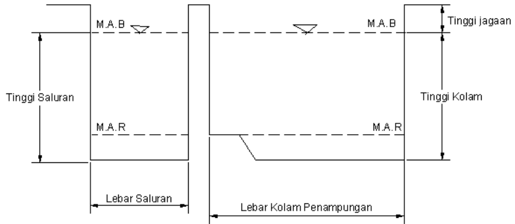
Gambar 2.6 Potongan I - I
