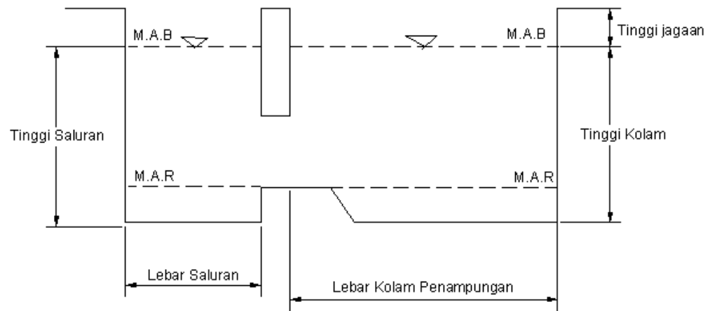
Gambar 2.7 Potongan II - II
