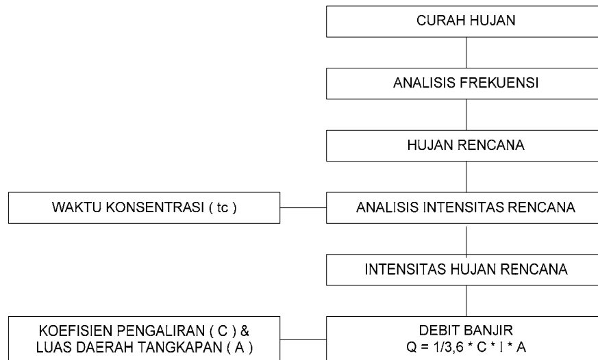
Gambar 2.8 Skema Analisa Hidrologi
