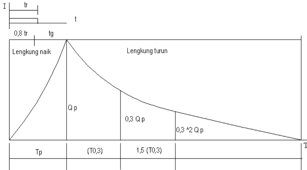
Gambar 2.4 Hidrograf Nakayasu
