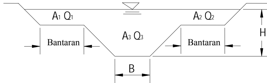
Gambar 2.3. Penampang Ganda
