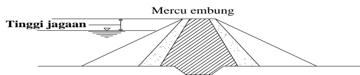
Gambar 2.12. Tinggi Jagaan Pada Mercu Embung
