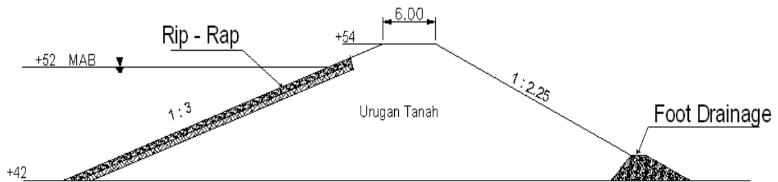
Gambar 2.9. Embung Type Urugan
