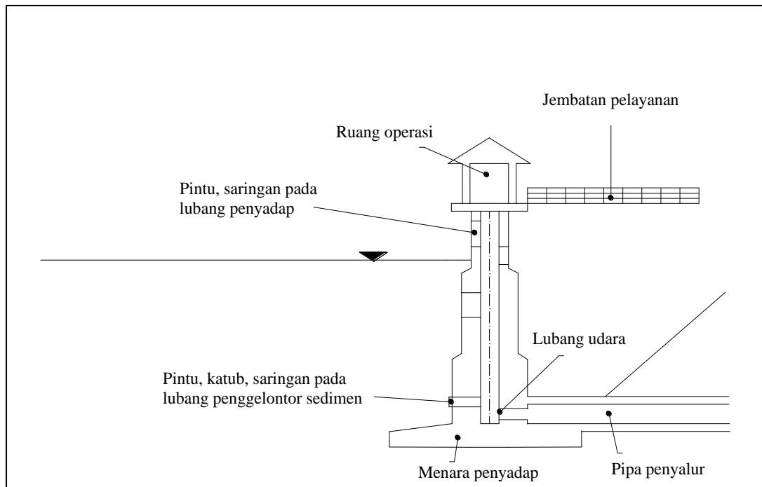
Gambar 2.32. Bangunan Penyadap Menara
