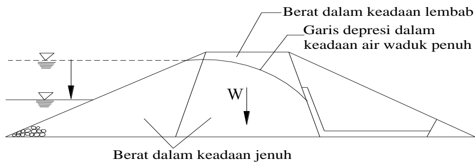
Gambar 2.15. Berat Bahan Yang Terletak Di Bawah Garis Depresi
