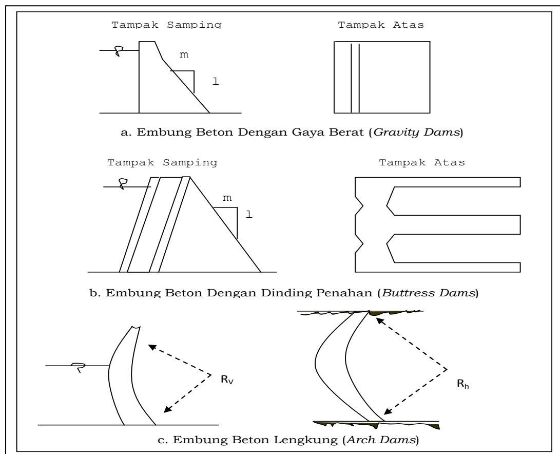
Gambar 2.10. Tipe-tipe embung beton
