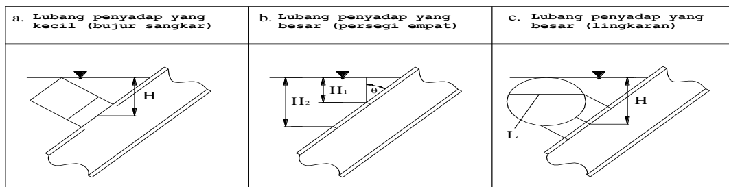
Gambar 2.31. Skema Perhitungan Untuk Lubang-Lubang Penyadap
