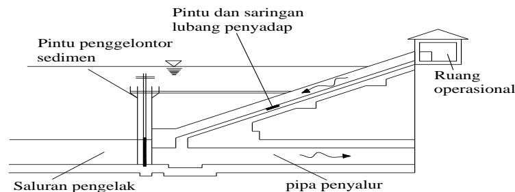
Gambar 2.30. Komponen Bangunan Penyadap Tipe Sandar
