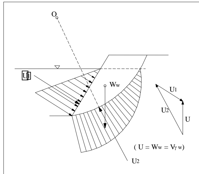
Gambar 2.17. Skema Pembebanan Yang Disebabkan oleh Tekanan Hidrostatik Yang Bekerja Pada Bidang Luncur
