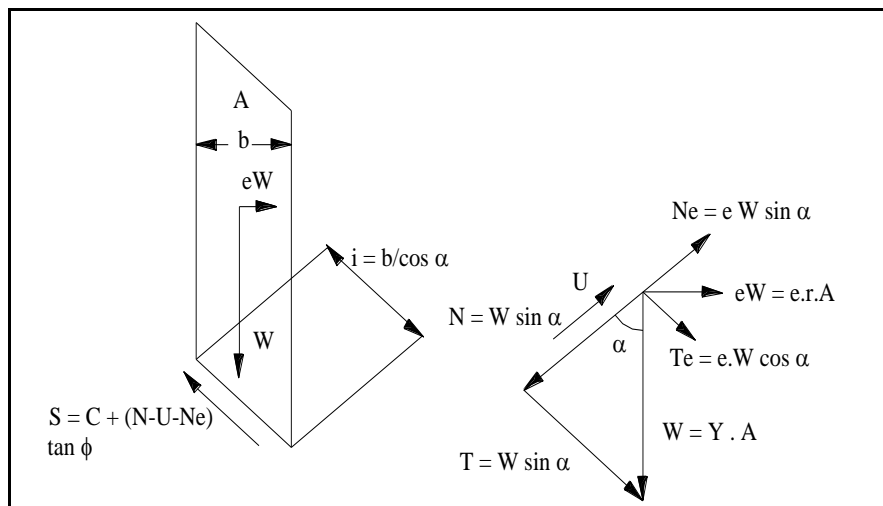
Gambar 2.18. Cara Menentukan Harga N dan T
