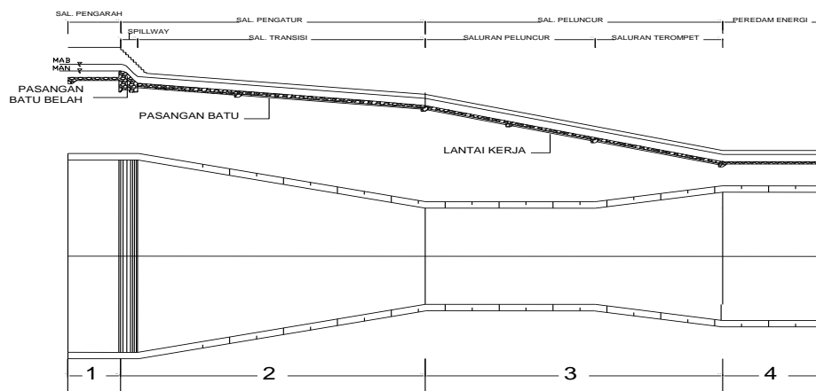
Gambar 2.24. Penampang Memanjang Bangunan Pelimpah
