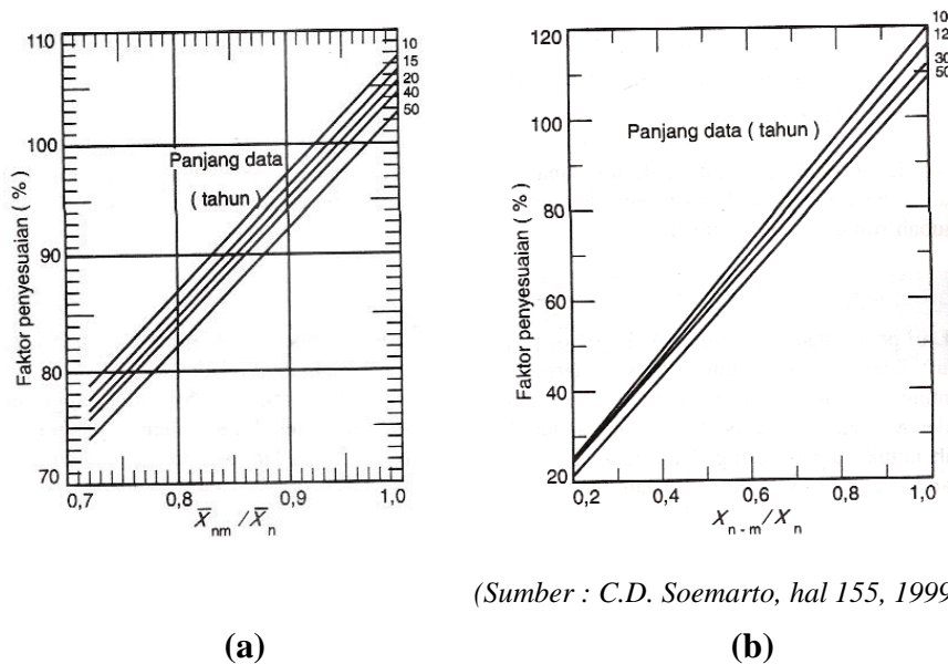
Gambar 2.3 Penyesuaian X_n dan S_n untuk data maksimum yang diamati
