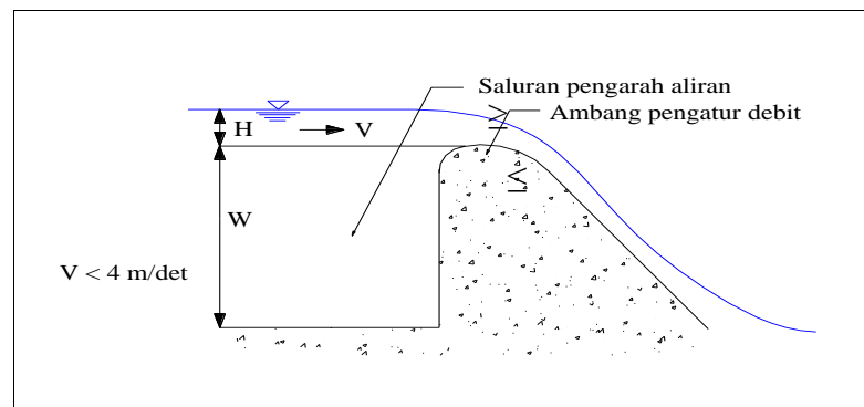
Gambar 2.23. Saluran Pengarah Aliran dan Ambang Pengatur Debit pada Sebuah Pelimpah
