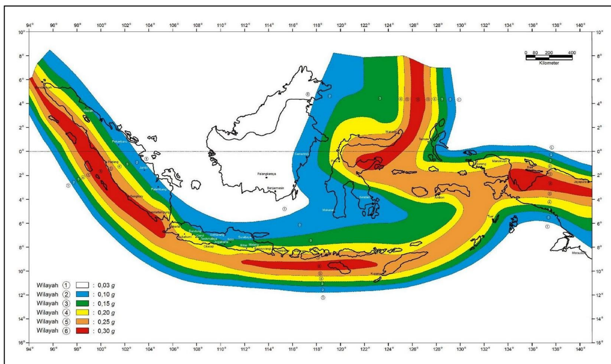
Gambar 2.14. Pembagian zone gempa di Indonesia
