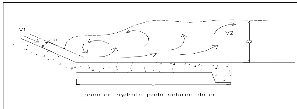
Gambar 2.26. Bentuk kolam olakan datar tipe I USBR
