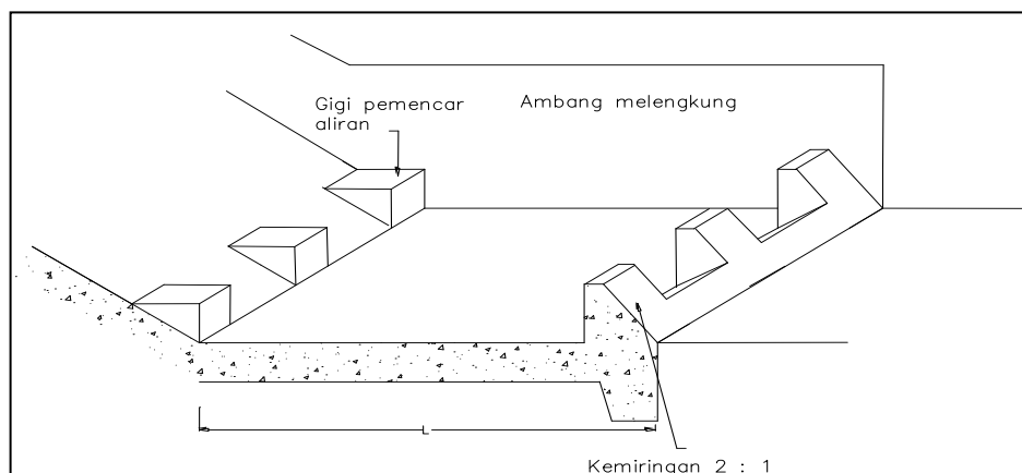
Gambar 2.27. Bentuk kolam olakan datar tipe II USBR
