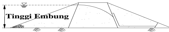
Gambar 2.11. Tinggi Embung
