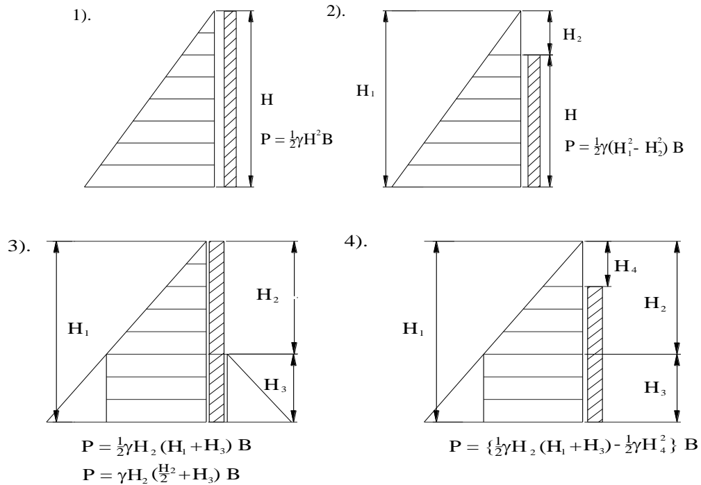
Gambar 2.33. Tekanan hidrostatis air
