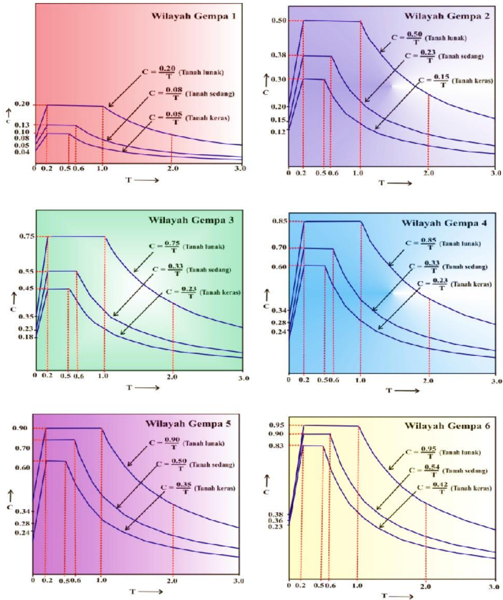
Gambar 2.3 Spektrum Respons
