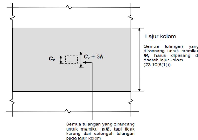
Gambar 2.9 Lokasi Tulangan Pada Konstruksi Pelat Dua Arah
