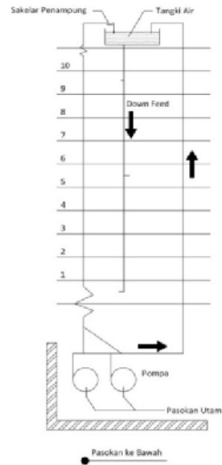
Gambar 2.1 Down Feed (Pasokan ke Bawah)
