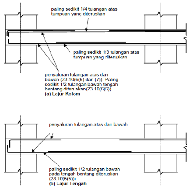
Gambar 2.10 Pengaturan Tulangan Pada Pelat
