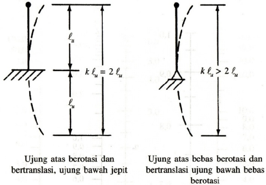
Gambar 2.5 Panjang Efektif Kolom Tumpuan Jepit dan Sendi
