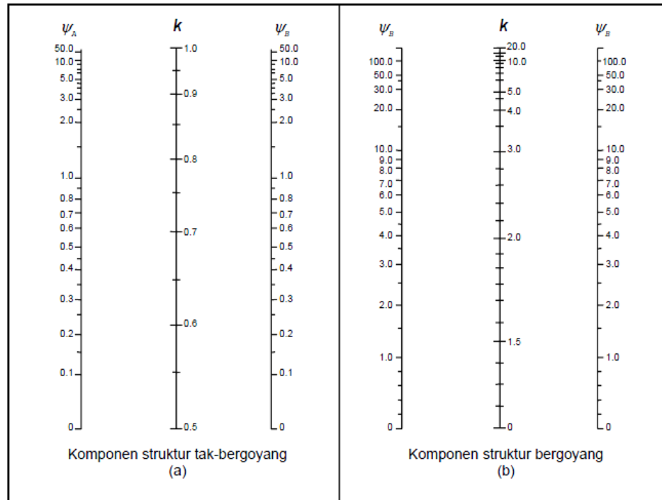
Gambar 2.6 Kurva Alinyemen untuk Portal Tak Bergoyang dan Portal Bergoyang
