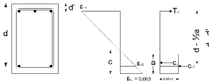
Gambar 2.8 Diagram Regangan dan Gaya-Gaya Dalam
