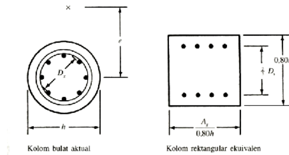
Gambar 2.4 Jenis Kolom Beton Bertulang
