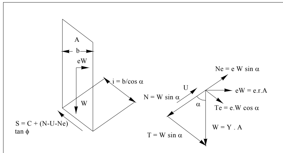
Gambar 3.18. Gambar Cara Menentukan Harga-Harga N dan T
