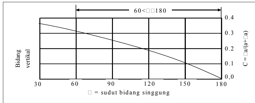
Gambar 3.17. Grafik hubungan antara sudut bidang singgung ( \alpha ) dengan \frac{\Delta a}{a + \Delta a}
