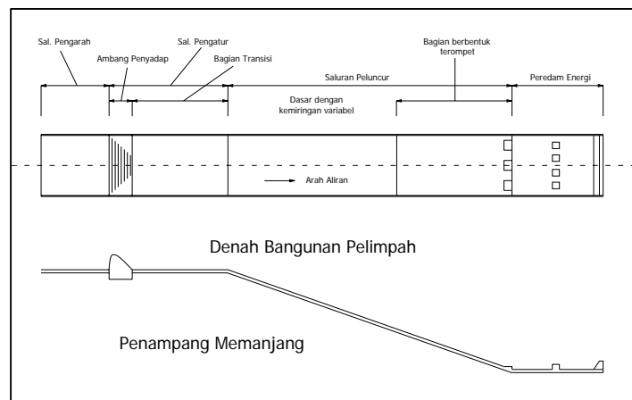
Gambar 3.10. Gambar Bangunan Pelimpah
