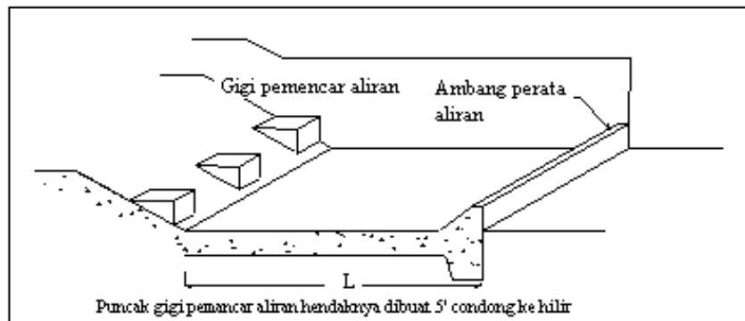
Gambar 3.13. Gambar Kolam Olakan Datar Tipe IV USBR
