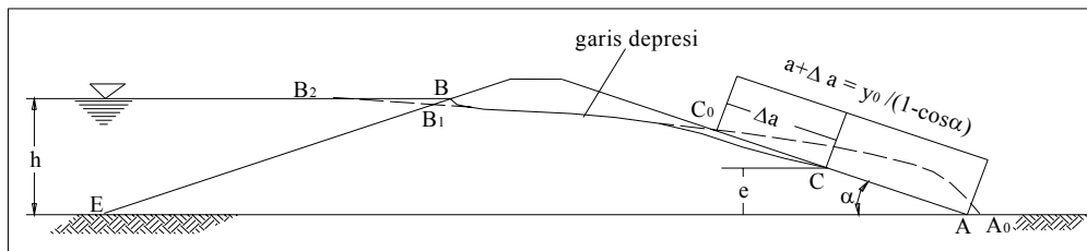
Gambar 3.16. Gambar Garis Depresi pada Embung Homogen (sesuai dengan garis parabola yang dimodifikasi)
