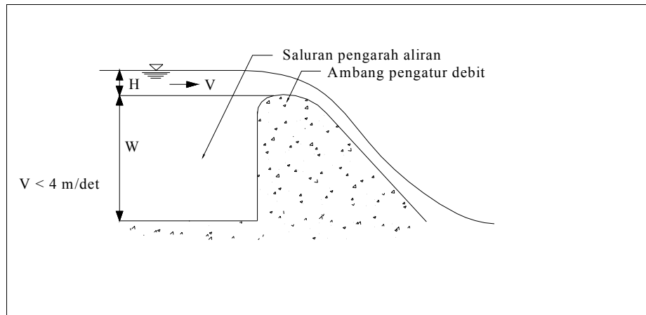
Gambar 3.9. Gambar Saluran Pengarah Aliran dan Ambang Pengatur Debit Pada Sebuah Pelimpah
