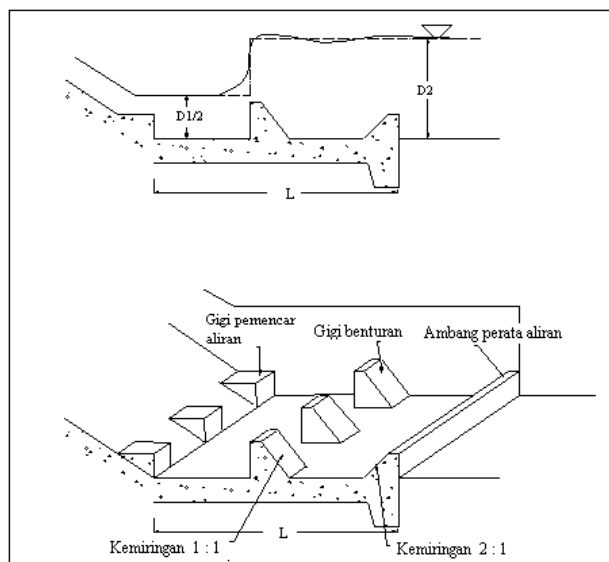
Gambar 3.12. Gambar Kolam Olakan Datar Tipe III USBR
