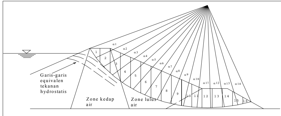
Gambar 3.19. Gambar Skema Perhitungan Bidang Lurur Dalam Kondisi Waduk Penuh Air
