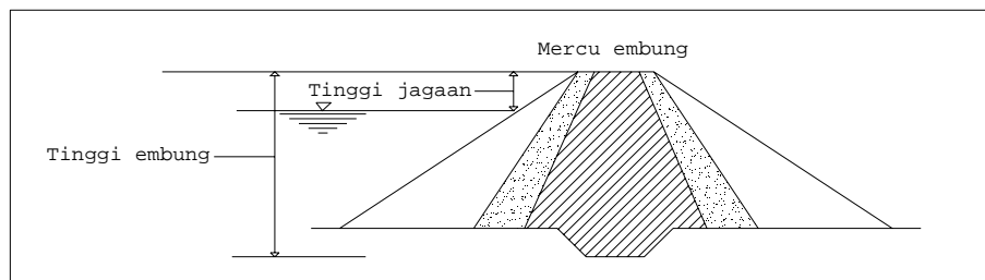
Gambar 3.14. Gambar Tinggi Embung dan Tinggi Jagaan Embung
