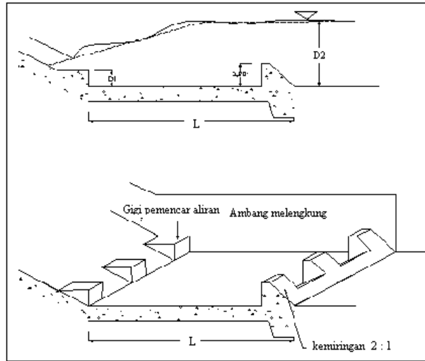
Gambar 3.11. Gambar Kolam Olakan Datar Tipe II USBR
