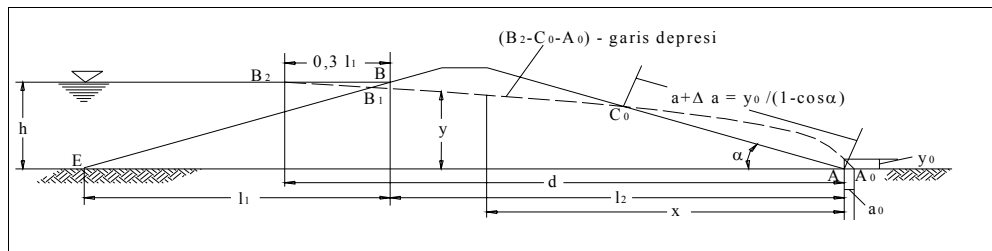
Gambar 3.15. Gambar Garis Depresi Pada Embung Homogen
