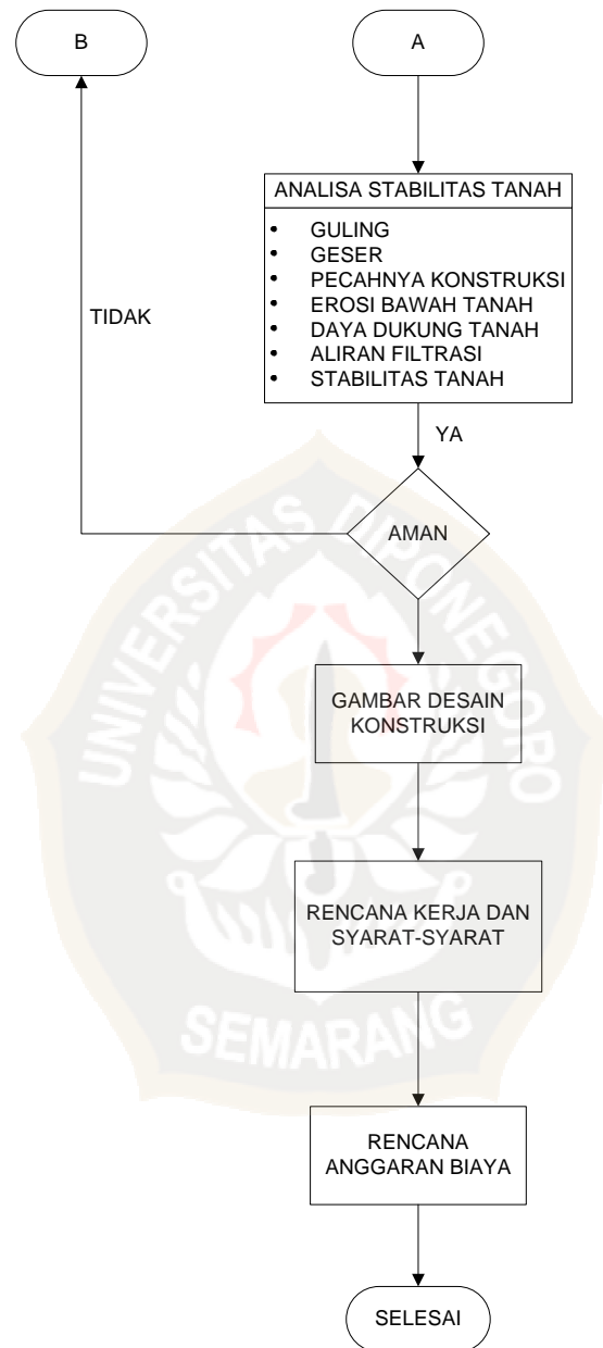
Gambar 3.1 Skema Urutan Perencanaan Embung Musuk
