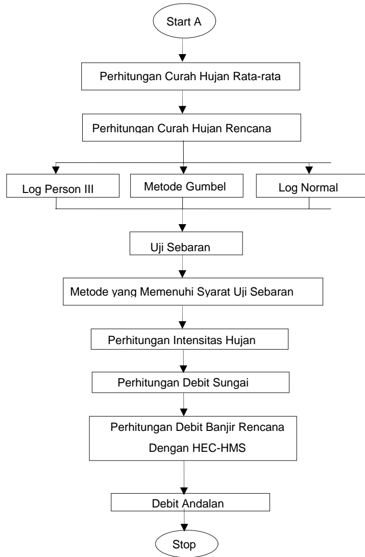
Gambar 3-2 Diagram Alir Analisis Hidrologi
