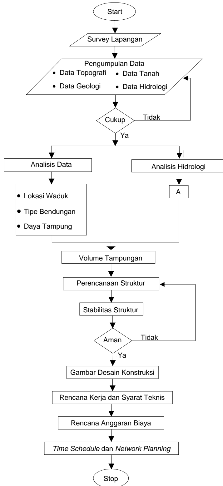
Gambar 3-1 Diagram Alir Rencana Kerja Tugas akhir
