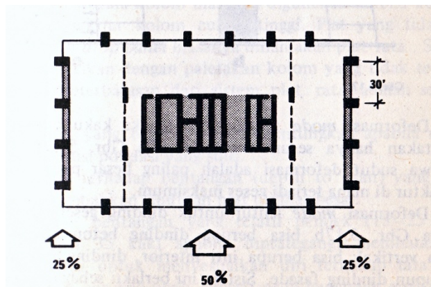
Gambar 2.14 Sistem interaksi rangka bersendi-Vierendeel-dinding geser
