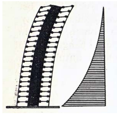
Gambar 2.13 Sistem rangka bersendi dinding geser
