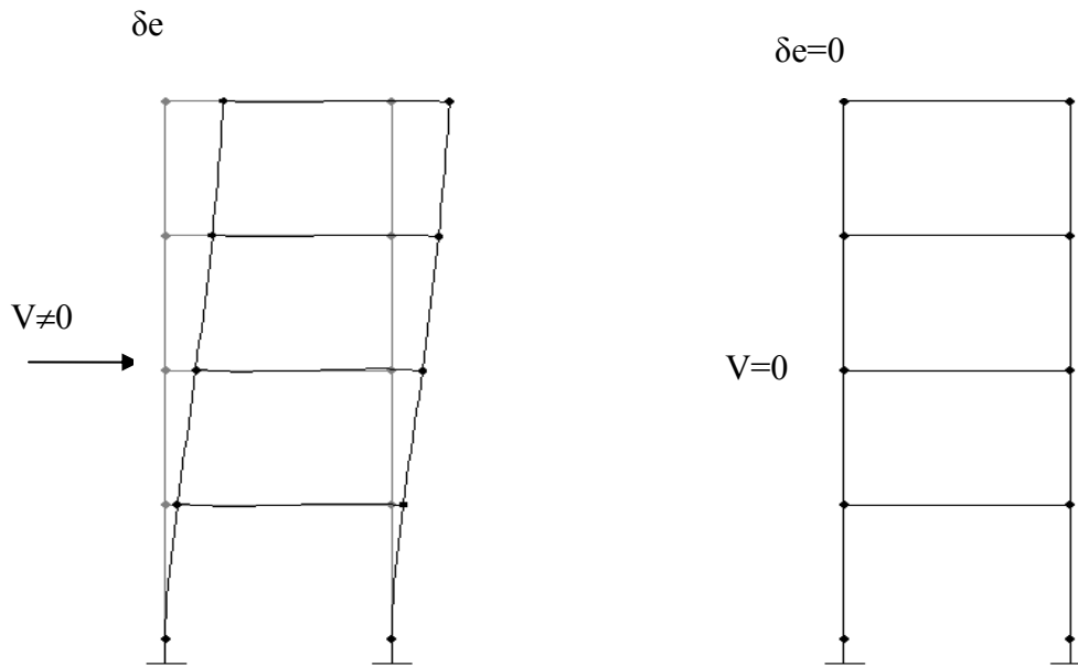
Gambar 2.18.a. Deformasi elastis pada struktur
