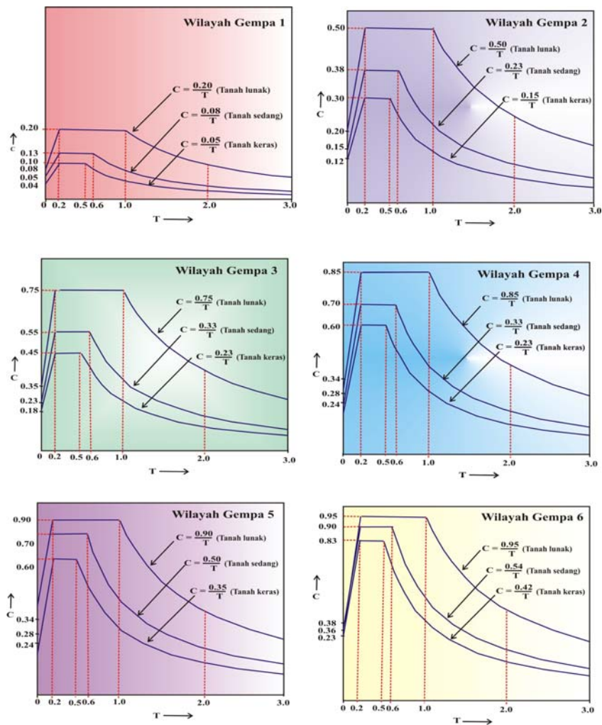
Gambar 2.17 Spektrum Respon untuk Masing-masing Daerah Gempa
