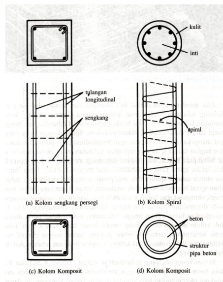
Gambar 2.26 Jenis – jenis Sengkang Pengikat
