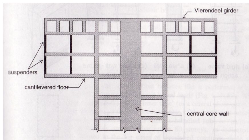
Gambar 2.7. Penggunaan suspender
