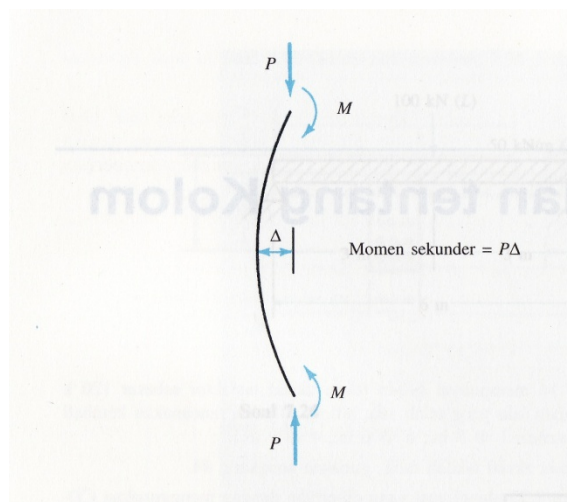
Gambar 2.23 Momen Sekunder yang terjadi pada kolom
