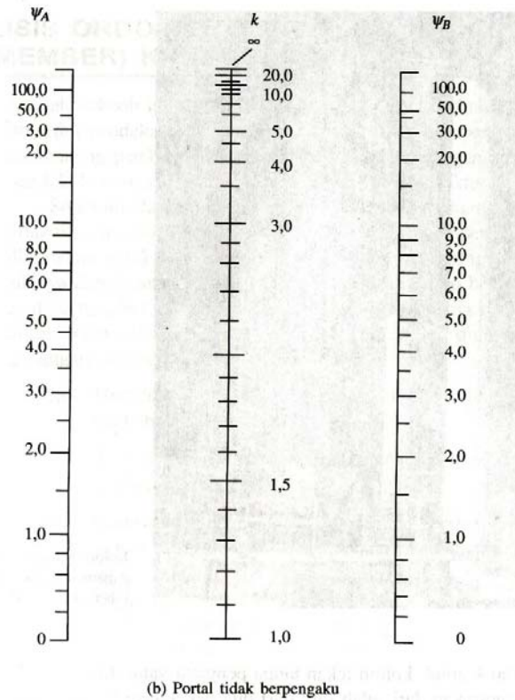
Gambar 2.24 Panjang Efektif untuk Portal Bergoyang
