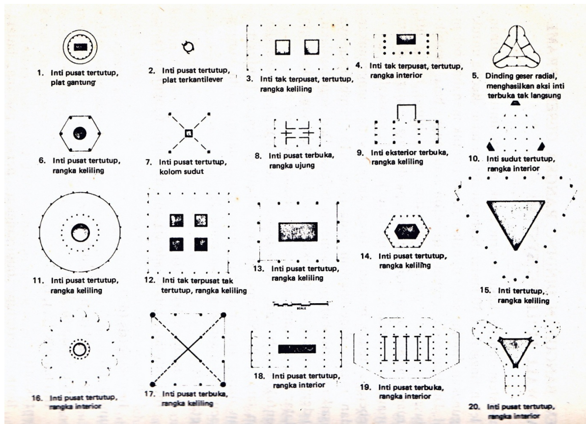
Gambar 2.12 Sistem Bangunan Dinding Rangka Geser
