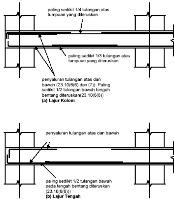
Gambar 2.21. Pengaturan Tulangan Pada Pelat
