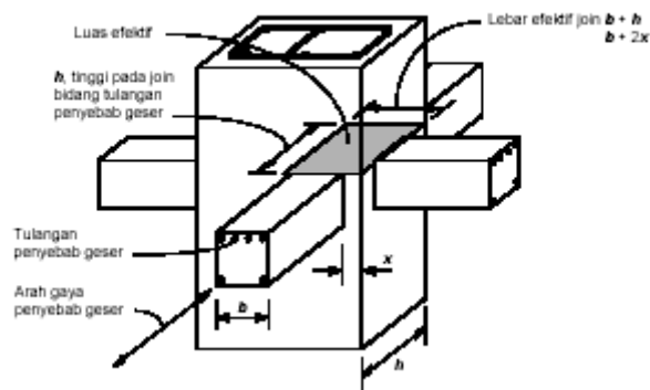
Gambar 2.29 Hubungan antara Balok dan Kolom
