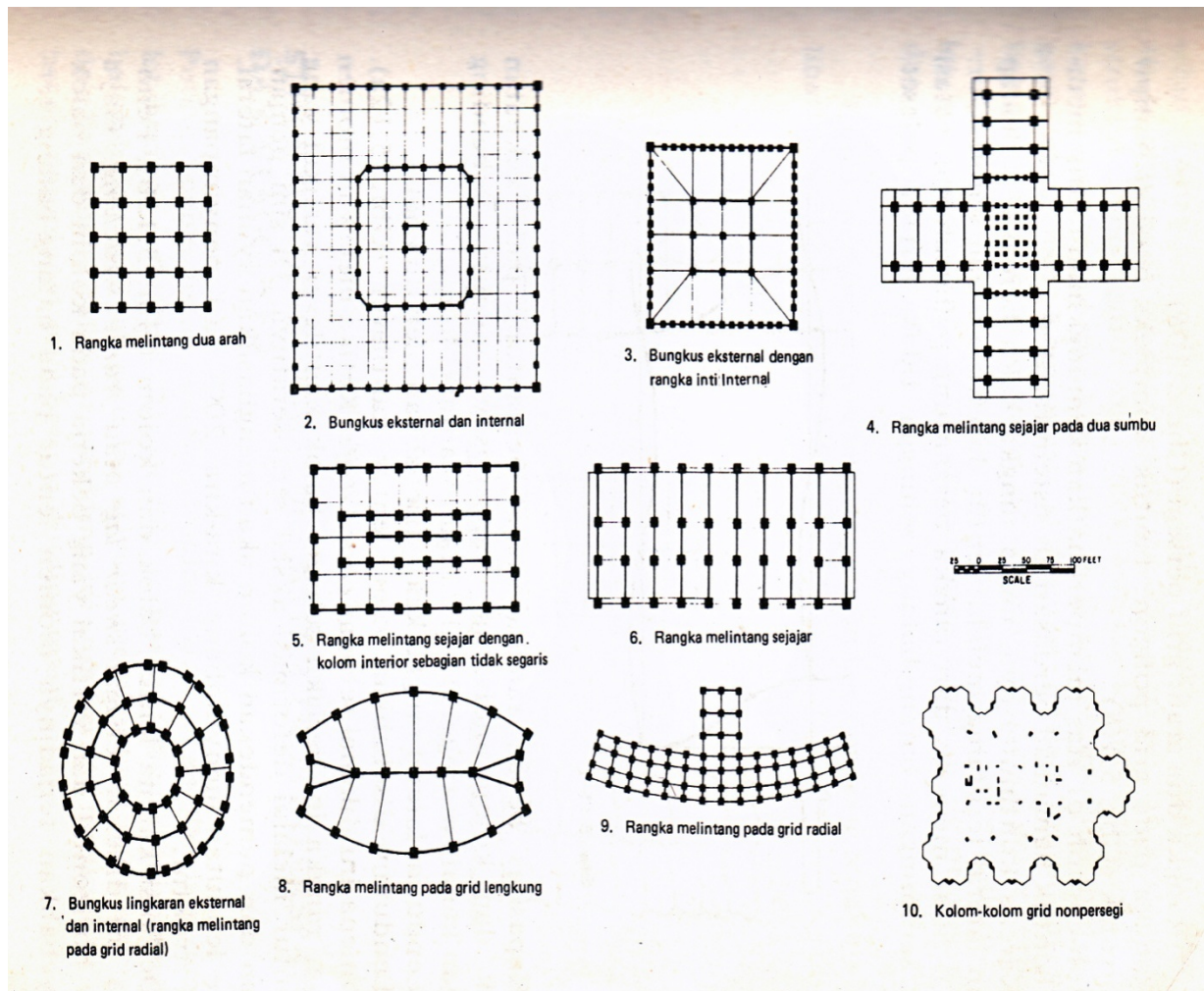
Gambar 2.9 Sistem Struktur Rangka Kaku
