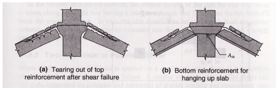
Gambar 2.28 Tulangan bawah pada drop panel
