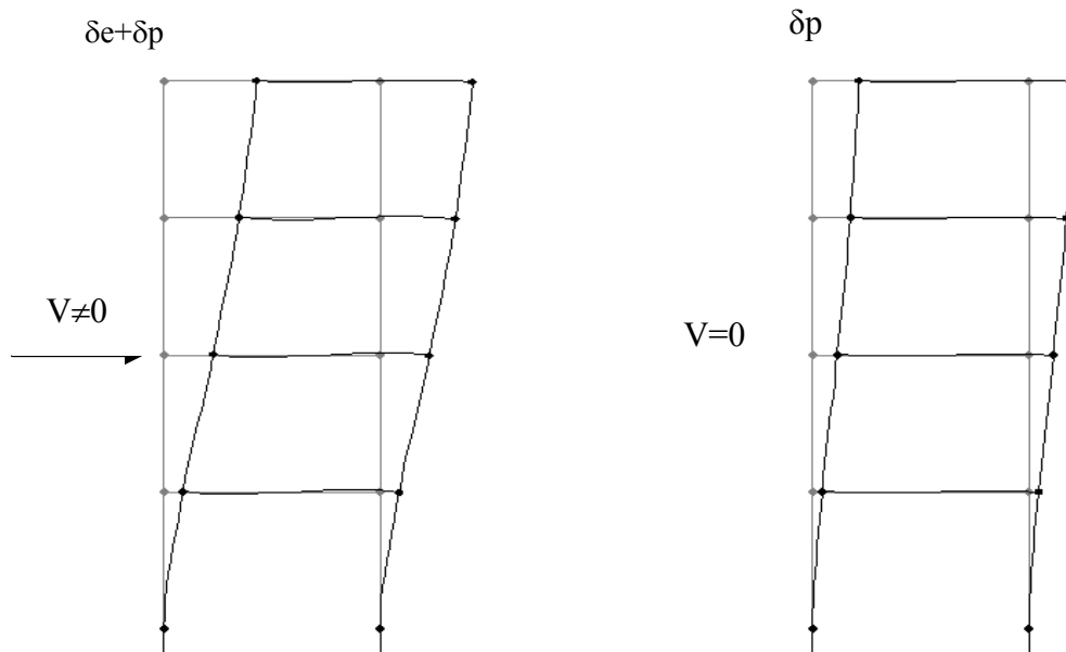
Gambar 2.18.b. Deformasi plastis (inelastis) pada struktur
