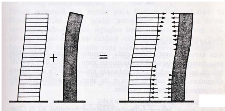
Gambar 2.15 Interaksi rangka kaku-dinding geser
