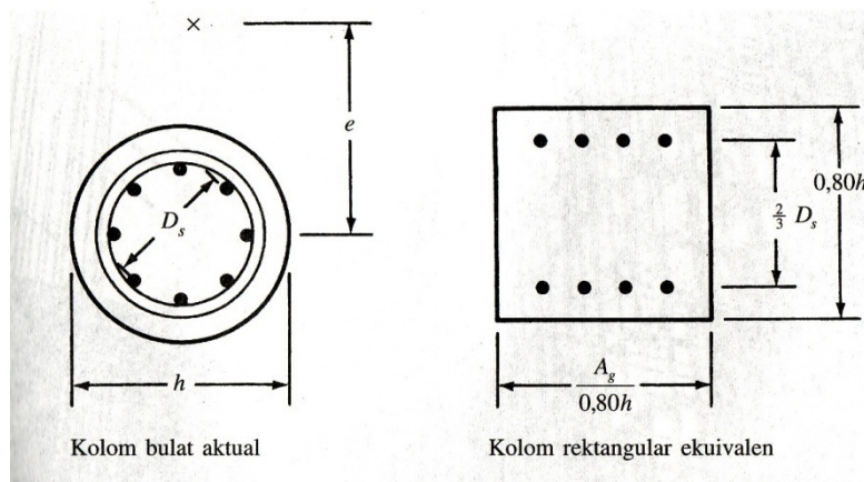
Gambar 2.22 Jenis – jenis Kolom Beton Bertulang
