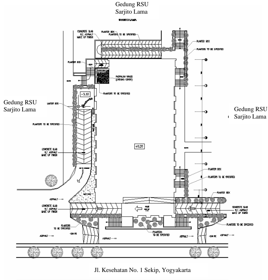
Gambar 1.1. Site Plan
