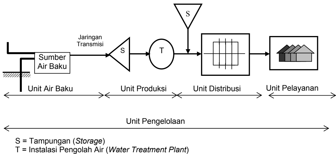
Gambar 3.1. Skematik Sistem Penyediaan Air Minum
