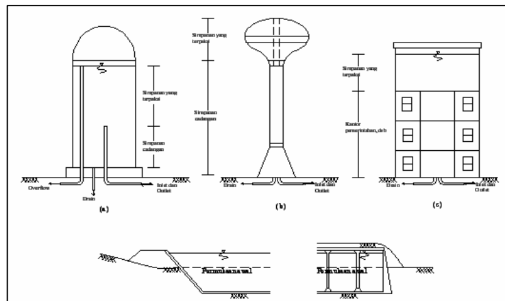
Gambar 3.10 Tipe-Tipe Reservoir Distribusi. (a) pipa tegak; (b) dan (c) tangki di atas permukaan tanah; (d) reservoir di permukaan tank
