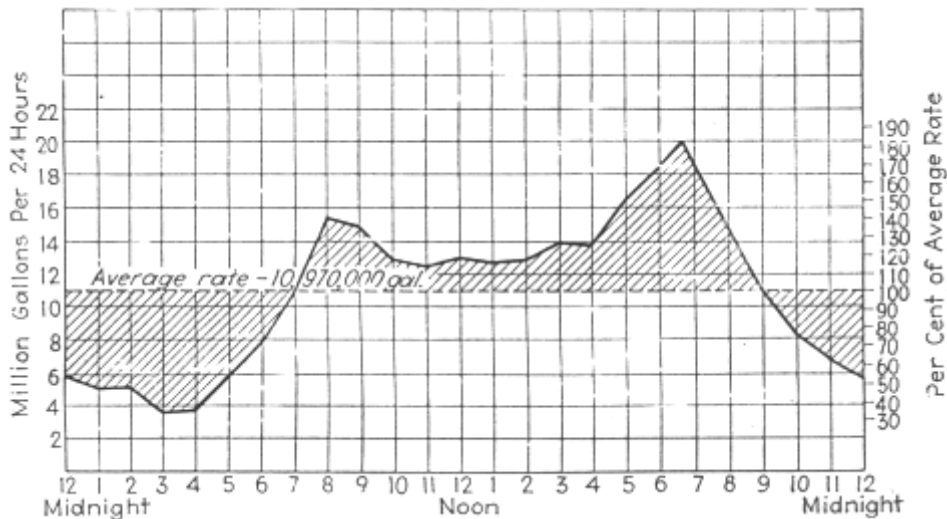
Gambar 3.2. Variasi Konsumsi Air Sepanjang Hari.
