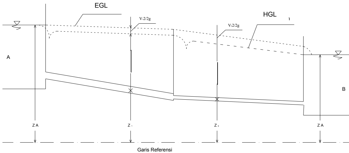
Gambar 3.8. Garis energi dan garis tekanan
