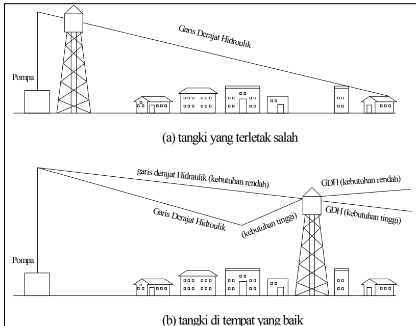
Gambar 3.9. Letak Tangki Tinggi Untuk Penampungan Air Sumber: Linsley (1996)
