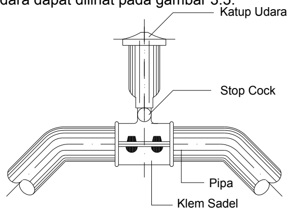
Gambar 3.5. Katup Udara
