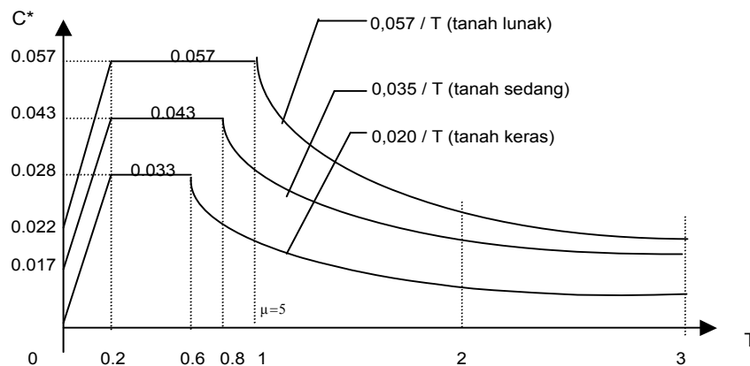
Gambar 2.1. Grafik Spektrum Respon Gempa
