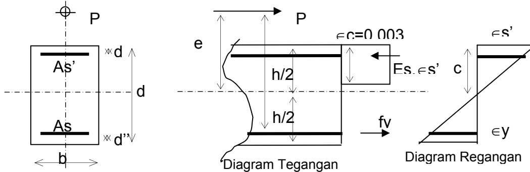
Gambar 2.7. Diagram Tegangan Regangan Penampang Balok Tertekan Eksentris Keadaan Balanced
