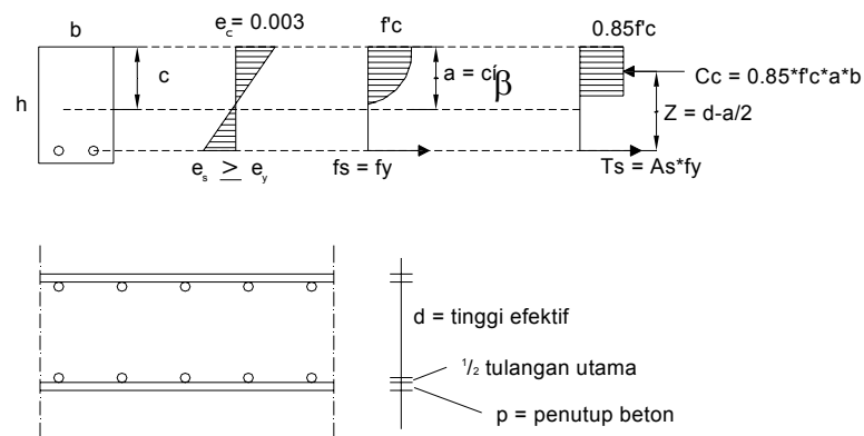
Gambar 2.5. Diagram Regangan – Tegangan Plat
