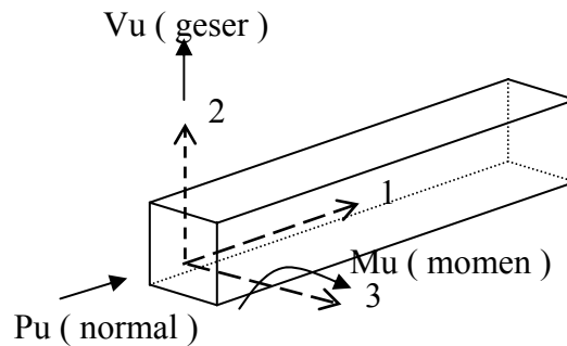
Gambar 2.6. Gaya-gaya pada elemen balok
