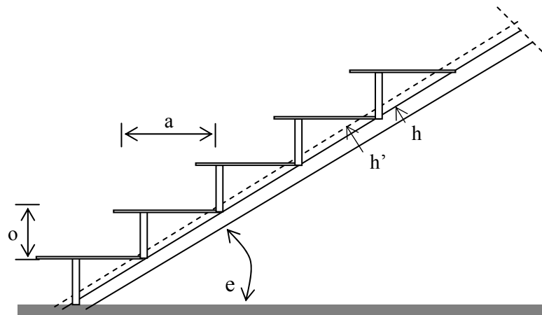
Gambar 2.9. Pendimensian Tangga
