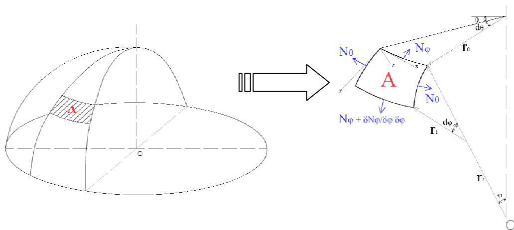
Gambar 2.2. Gaya yang terjadi pada Cangkang Kubah
