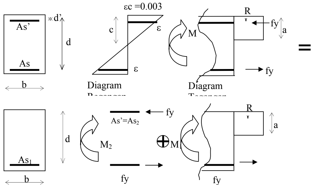
Gambar 2.8. Diagram Tegangan-Regangan Penampang Balok Dengan Tulangan Dobel
